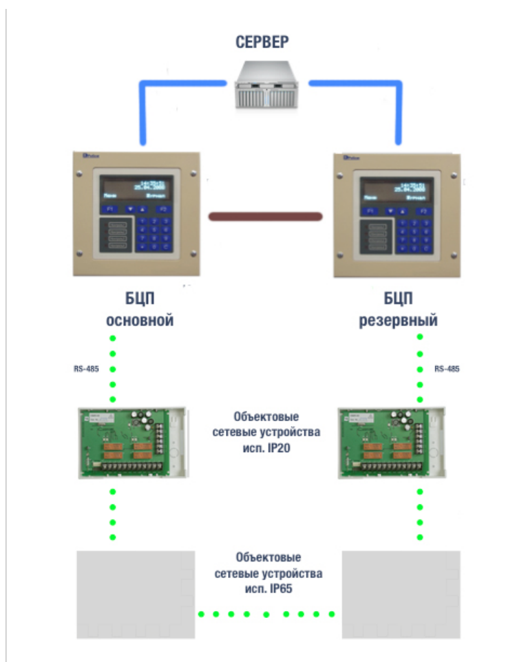
Рис. 1. Схема резервирования БЦП
