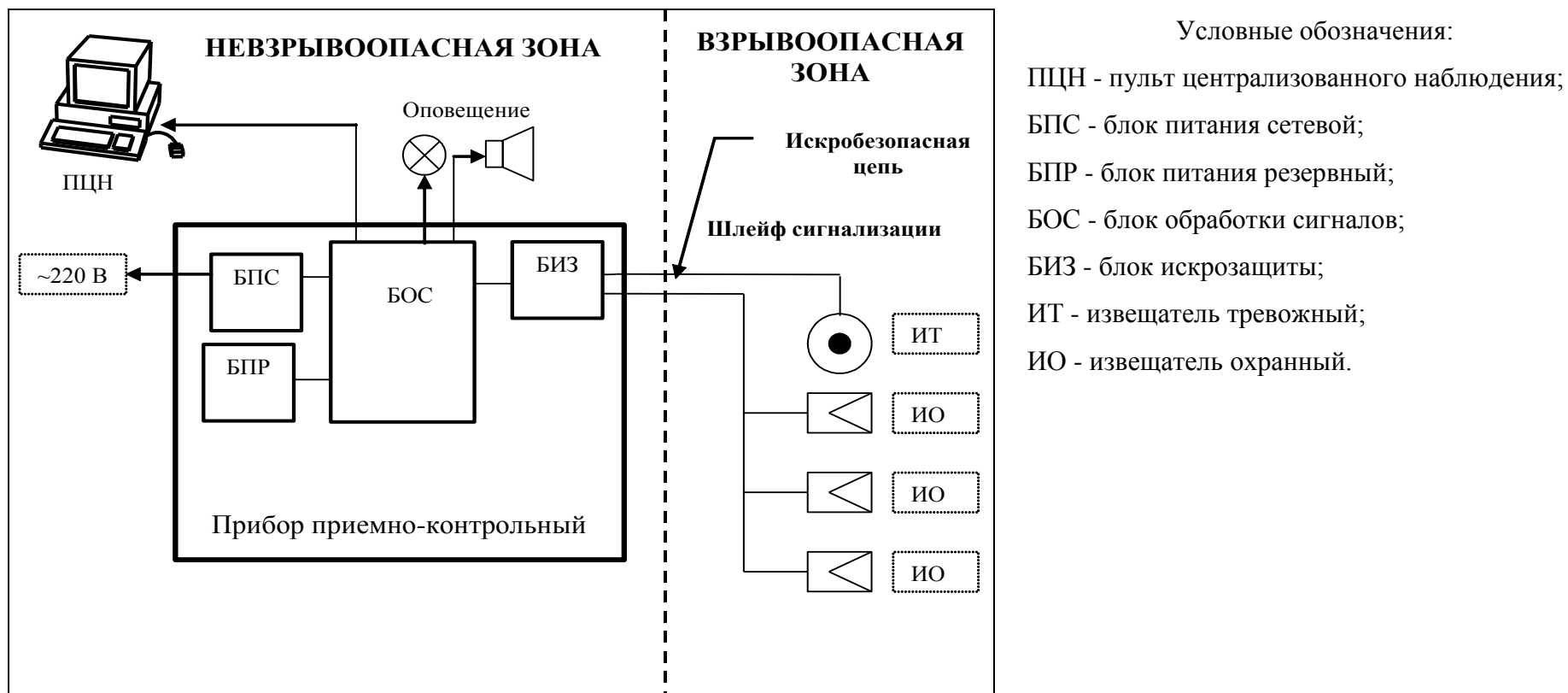
Рис.6.2 Оборудование объекта с взрывоопасными зонами.
