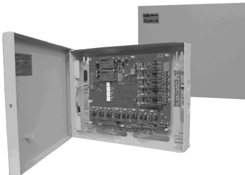
Рис. 6.3 Блок расширения шлейфов сигнализации.
