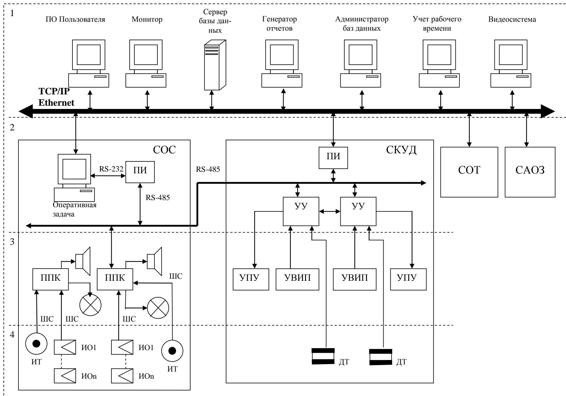
Рис. 2.1. Обобщенная структура ИСБ на основе локальных сетей.
