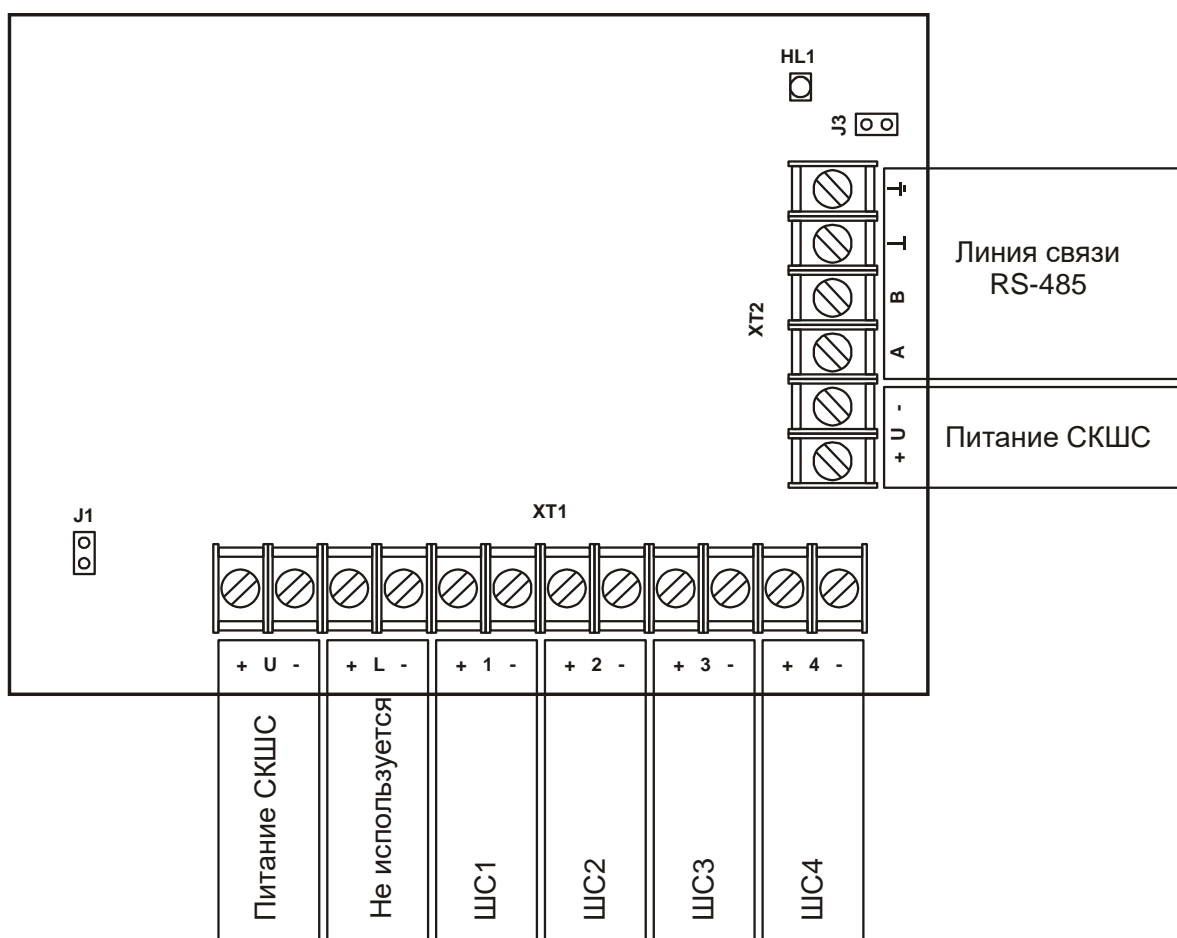
Рис. 17 Подключение СКШС
