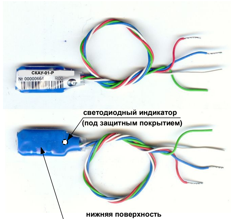
Рис. 2 Проводники подключения
