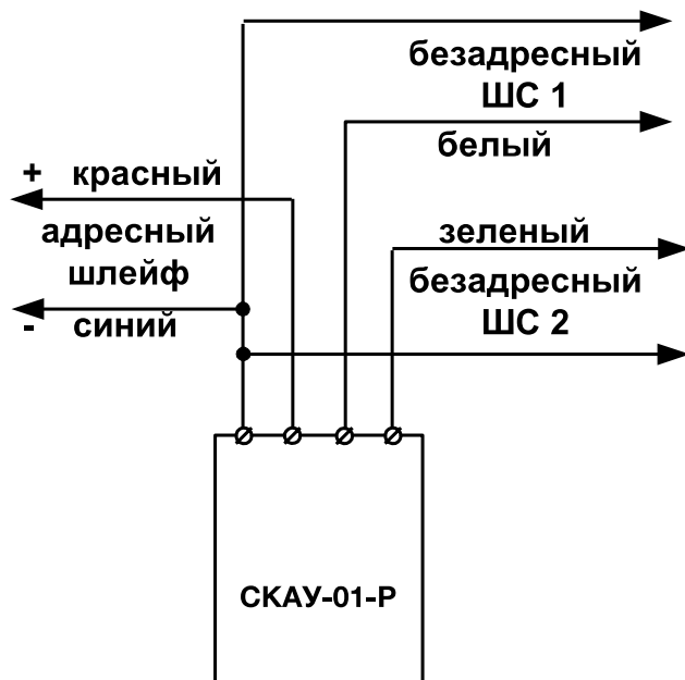
Рис. 5 Подключение двух шлейфов.
