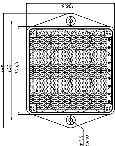
Рефлектор ДПРМ.203625.005 (тип СМ) (см. табл.1)
