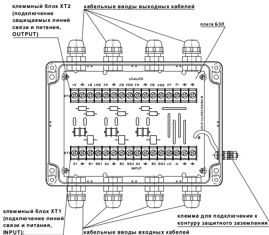
Рис. 1 БЗЛ-01, БЗЛ-04 (вид без крышки корпуса)
