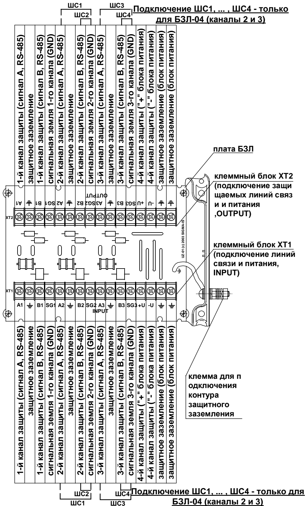
Рис. 3 Плата БЗЛ-01, БЗЛ-04
