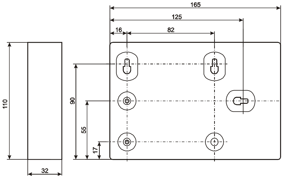
Рис. 24 Габаритные и присоединительные размеры (исполнение IP20)
