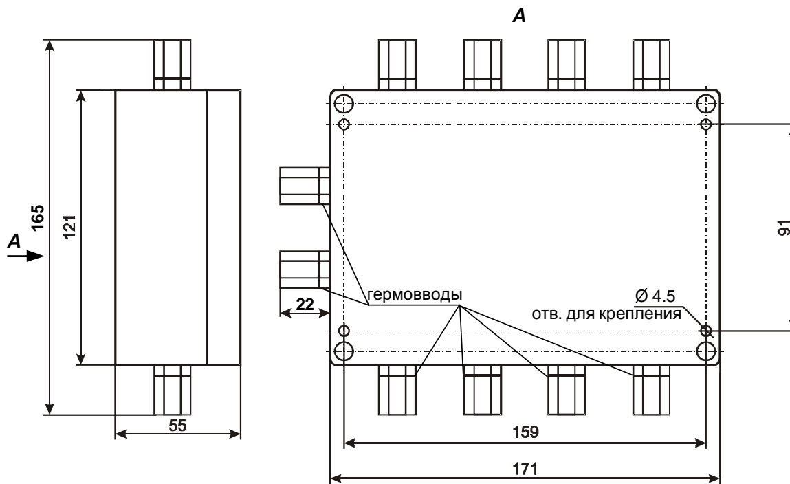
Рис. 25 Габаритные и присоединительные размеры (исполнение IP65)
