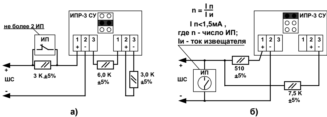
Рис. 12 Пожарный ШС с включением ручного ИП типа ИПР-3 СУ
