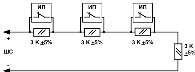
Рис. 9 Пожарный ШС с пассивными ИП (при срабатывании одного ИП формируется извещение «Внимание», более одного - «Пожар»)
