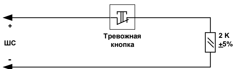
Рис. 7 Тревожный ШС
