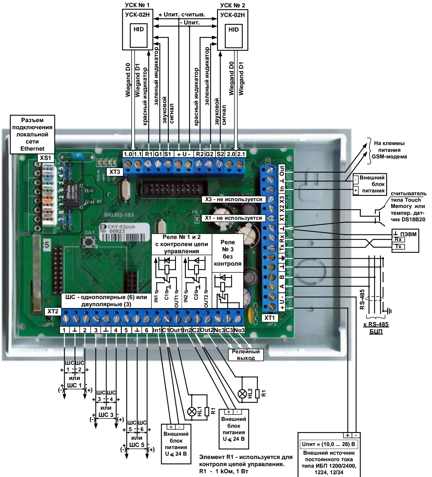
Рис. 3 Подключение СКУ
