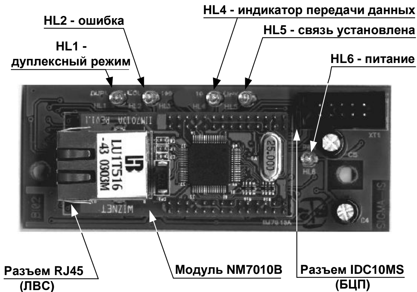
Рис. 3. Конструкция БИ-03.
