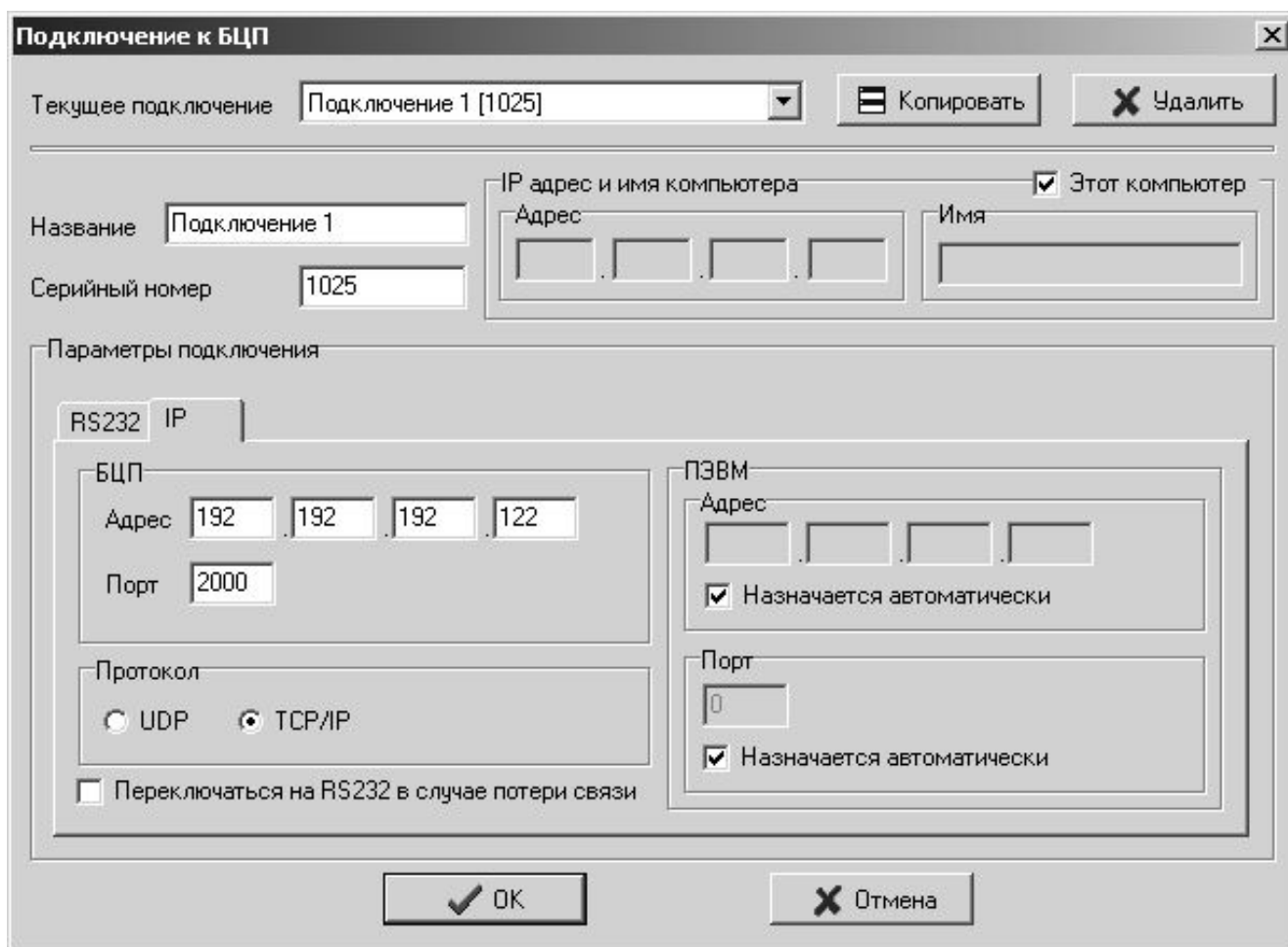
Рис. 9. Настройка подключения к БЦП в программе “Рубеж Консоль”.
