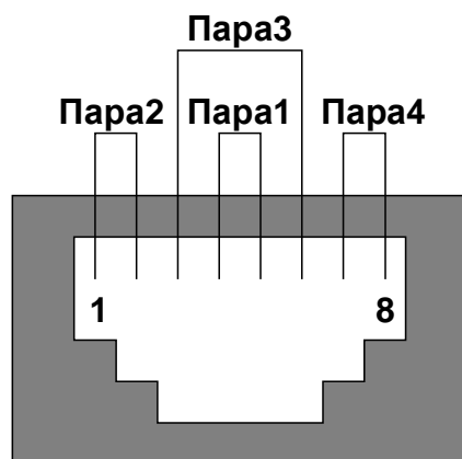
Рис. 6. Разводка RJ-45
