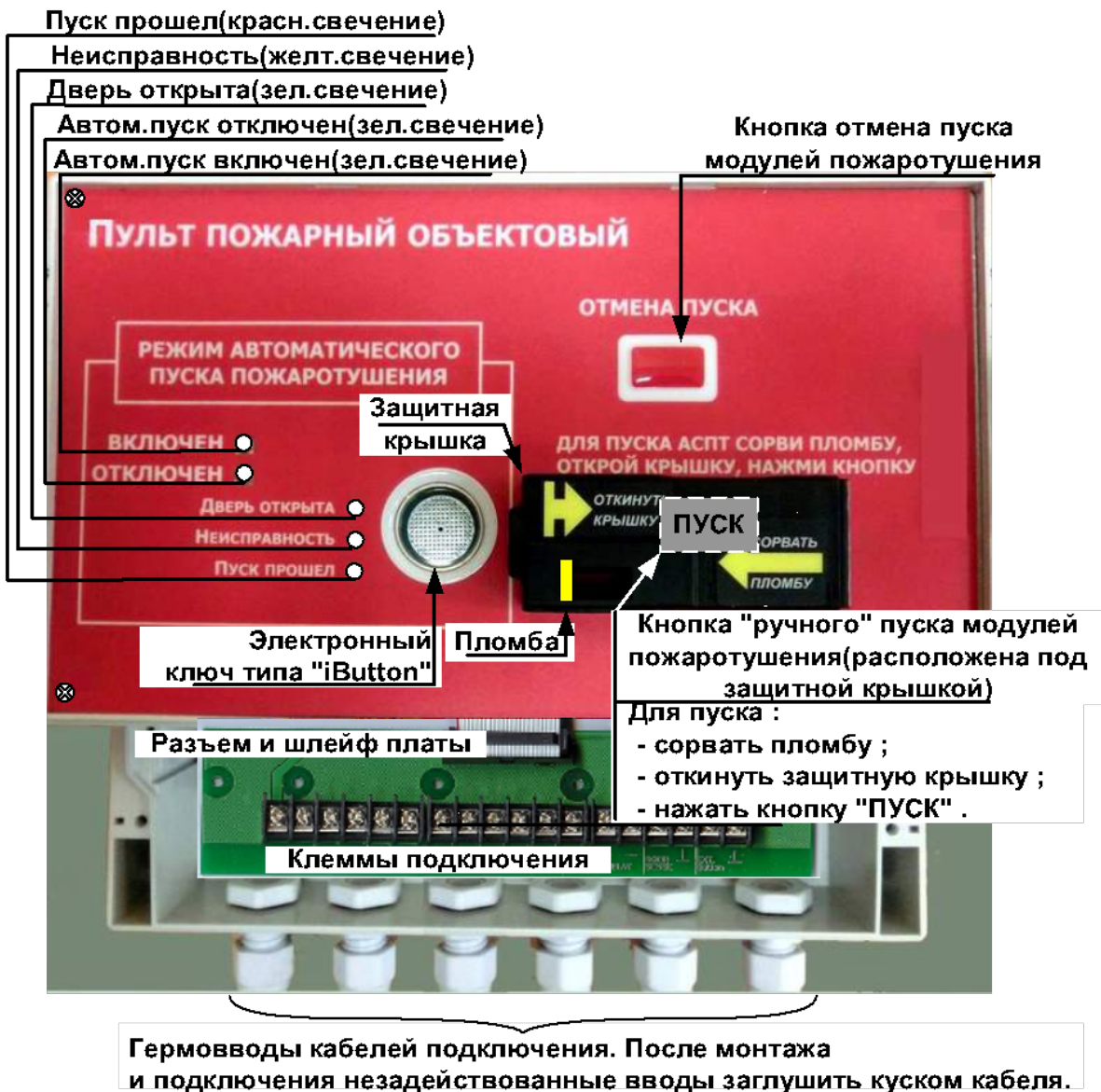
Рис. 2 Внешний вид ППО с открытой крышкой
