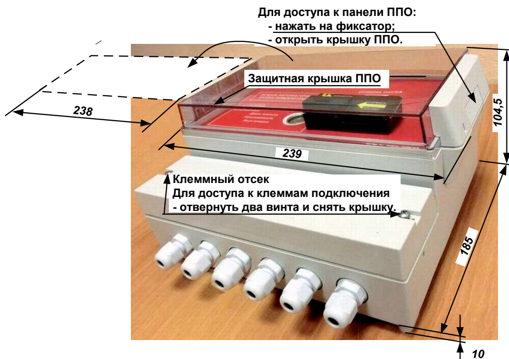
Рис. 1 Внешний вид ППО-01 исп.08. Габаритные размеры.
