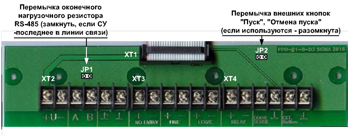
Рис. 3 Расположение элементов на плате подключения
