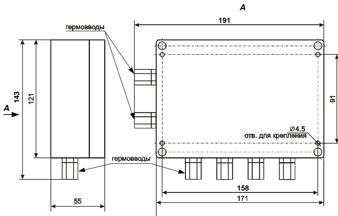
Рис. 4 Габаритные и присоединительные размеры КА2 исп.08, IP20
