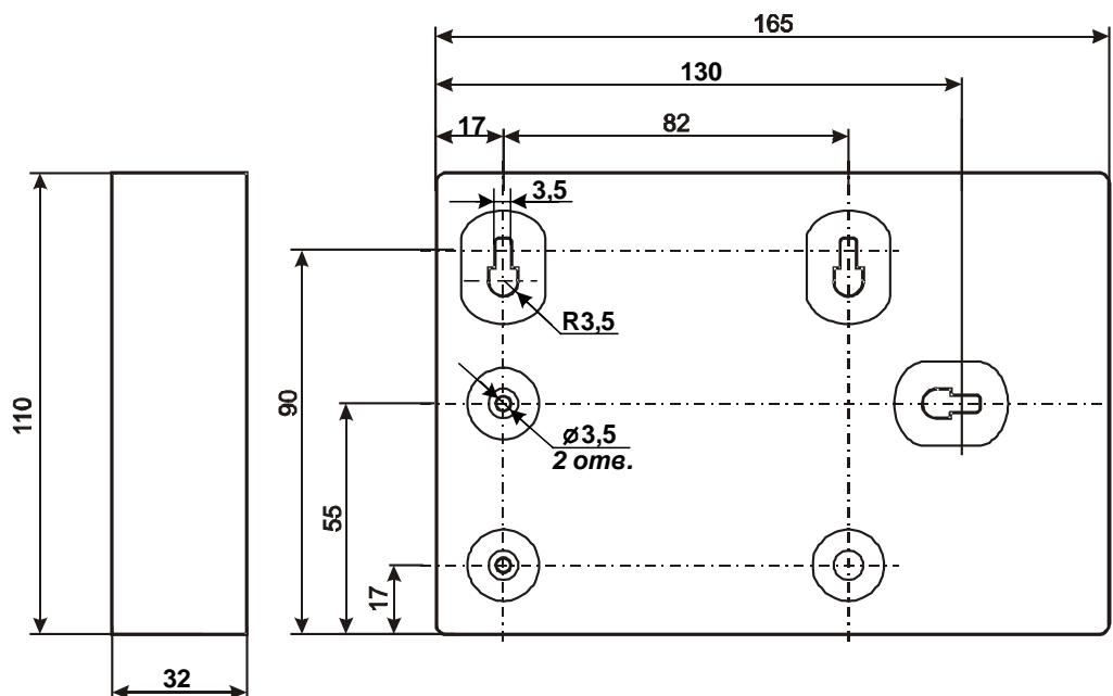
Рис. 4 Габаритные и присоединительные размеры КА2 исп.08, IP20
