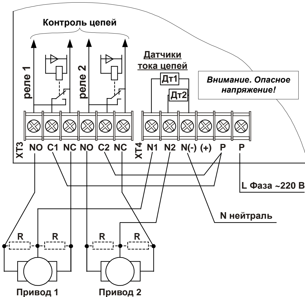
Рис. 6 Подключение 2-х реверсивных приводов переменного тока типа Белимо.
