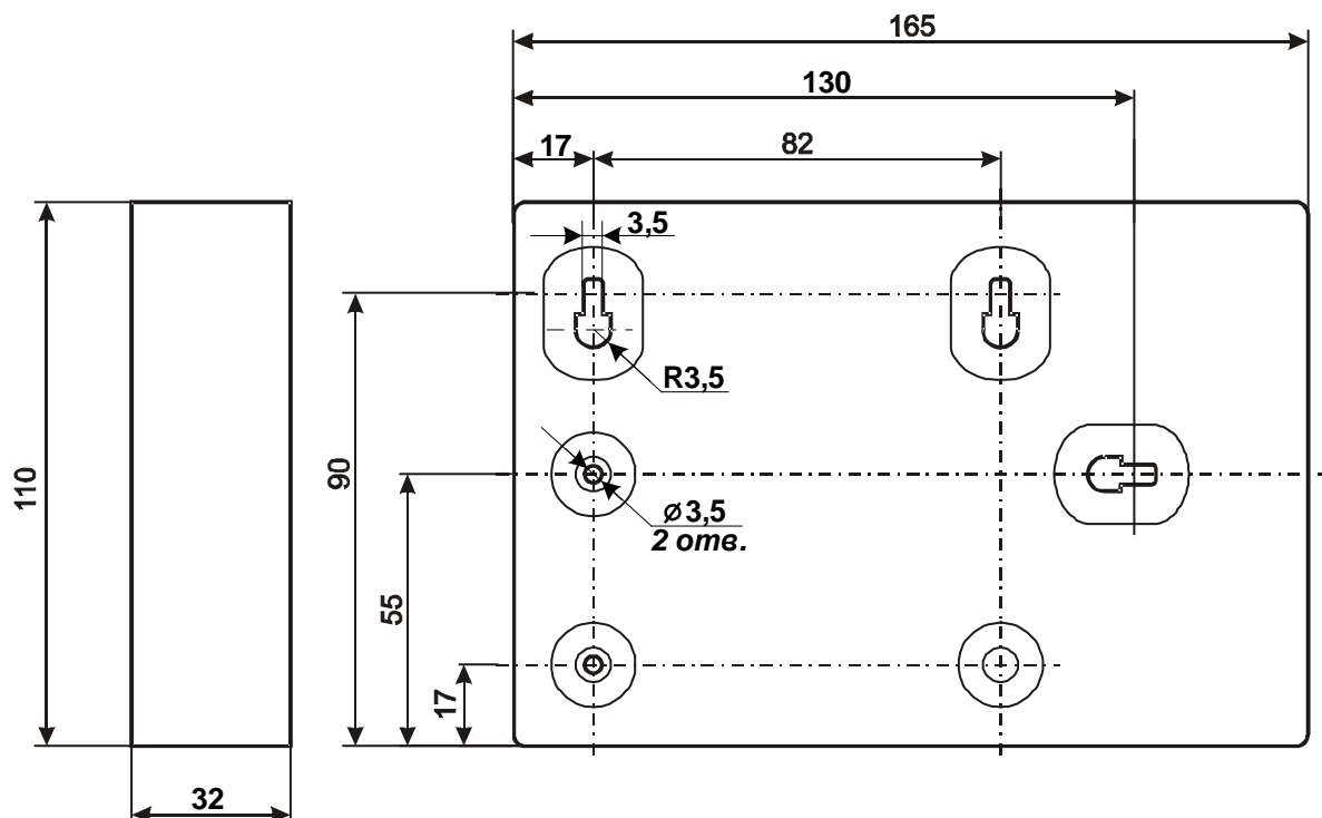
Рис. 2 Габаритные и присоединительные размеры корпуса ИСМ220 исп.08-4 (IP20)
