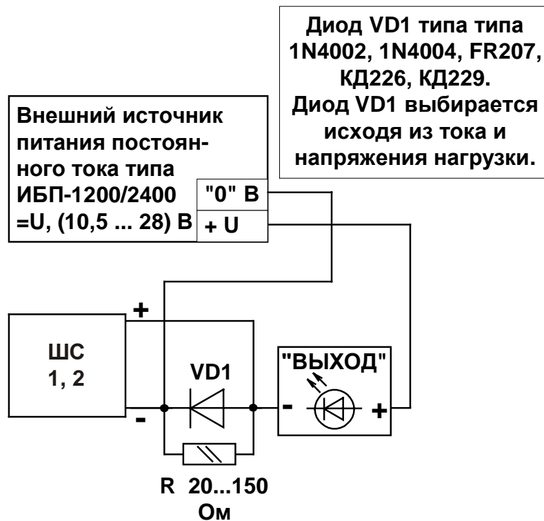
Рис. 10 Подключение светового оповещателя
