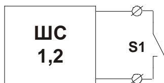
Схема 6 Подключение НР контактов без контроля целостности линии связи.
