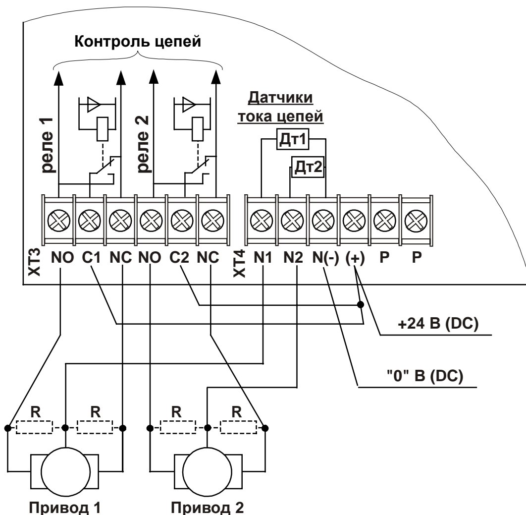
Рис. 7 Подключение 2-х реверсивных приводов типа Белимо постоянного тока 10..40 В
