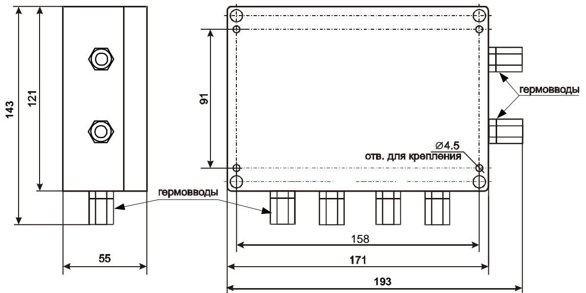
Рис. 3 Габаритные и присоединительные размеры корпуса ИСМ220 исп.4(08)К (IP65)
