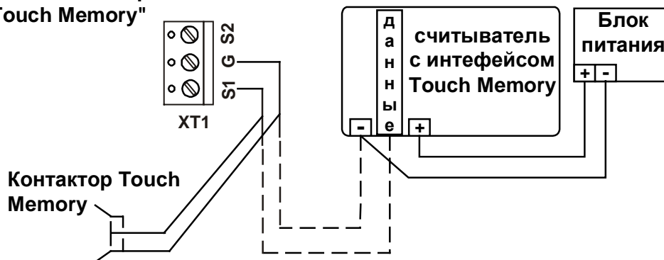
Рис. 11 Подключение контактора или считывателя(пунктиром) Touch Memory
