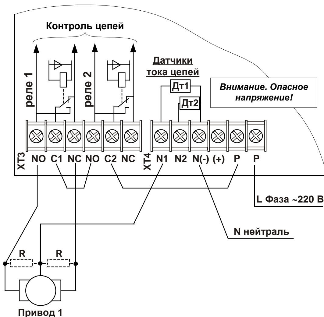
Рис. 8 Подключение 1-го реверсивного привода переменного тока типа Белимо с возможностью отключения напряжения
