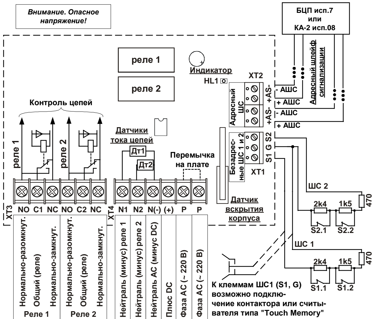
Рис. 1 Внешний вид, расположение элементов, подключение ИСМ220
