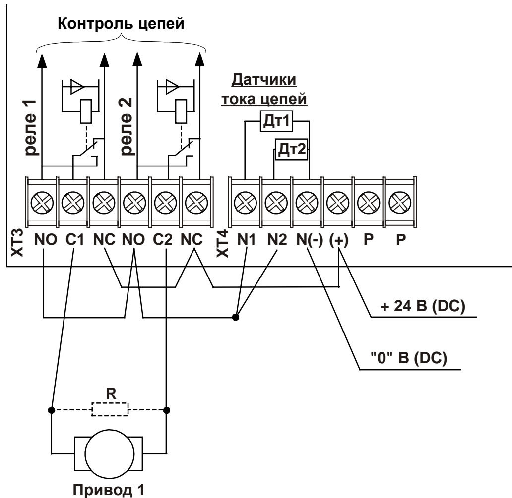
Рис. 9 Подключение реверсивного привода с переполюсовкой постоянного тока 10..40 В
