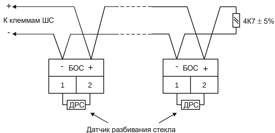
Рис. 12 Схема включения ИО «Окно»
