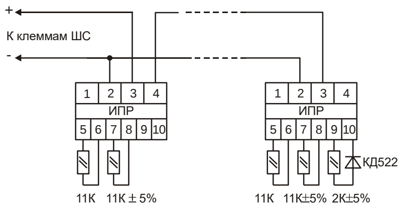
Рис. 6 Схема включения ручных ИП (ИПР и т. п.)
