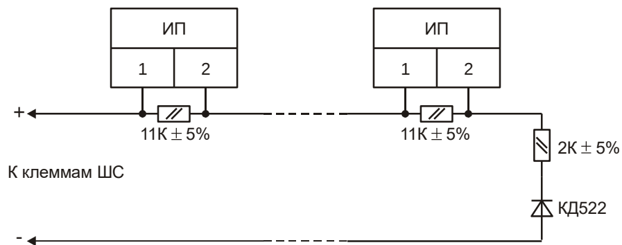
Рис. 4 Схема включения ИП с нормально-замкнутыми контактами (ИП103-4/1, ИП105-2/1 и т.п.)
