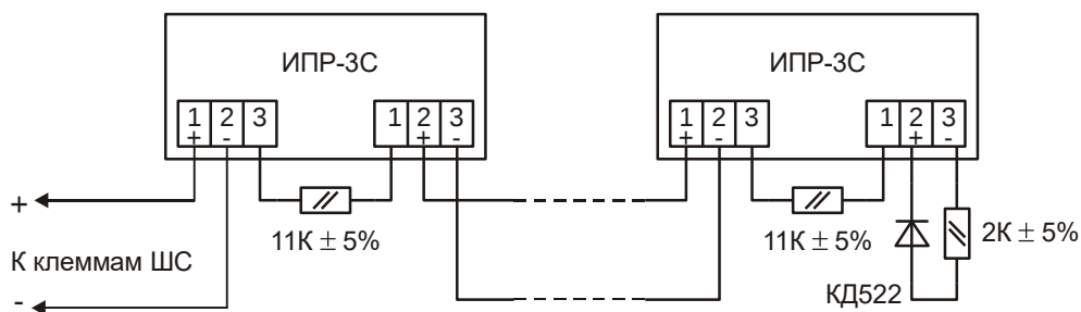
Рис. 6 Схема включения ручных ИП (ИПР и т. п.)
