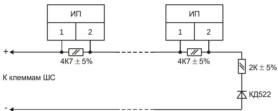
Рис. 8 Схема включения ИП с нормально-замкнутыми контактами (ИП105-2/1 и т. п.)
