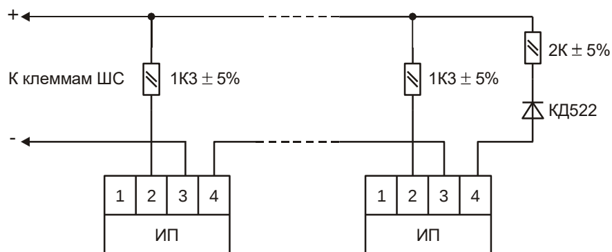
Рис. 9 Схема включения ИП с нормально-разомкнутыми контактами (ИП-212-5М и т.п.)
