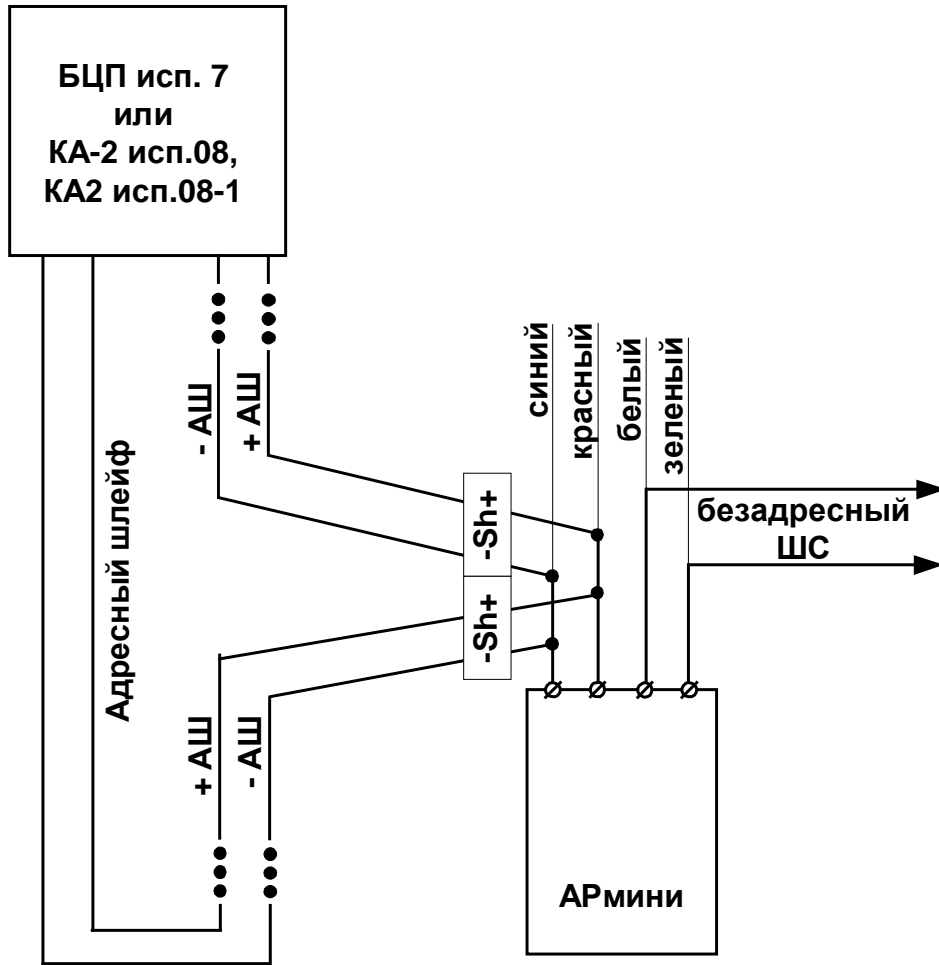
Рис. 2 Подключение устройства с одним ШС
