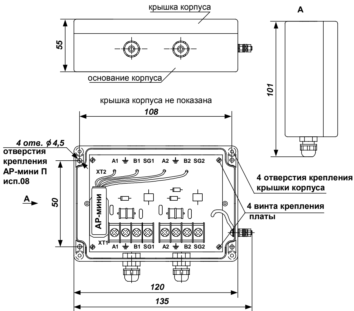
Рис. 11 Конструкция АРмини-П исп.08
