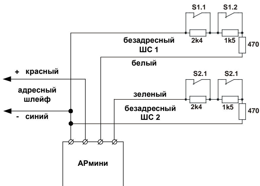
Рис. 5 Пример подключения 4-х извещателей с НЗ контактами.
