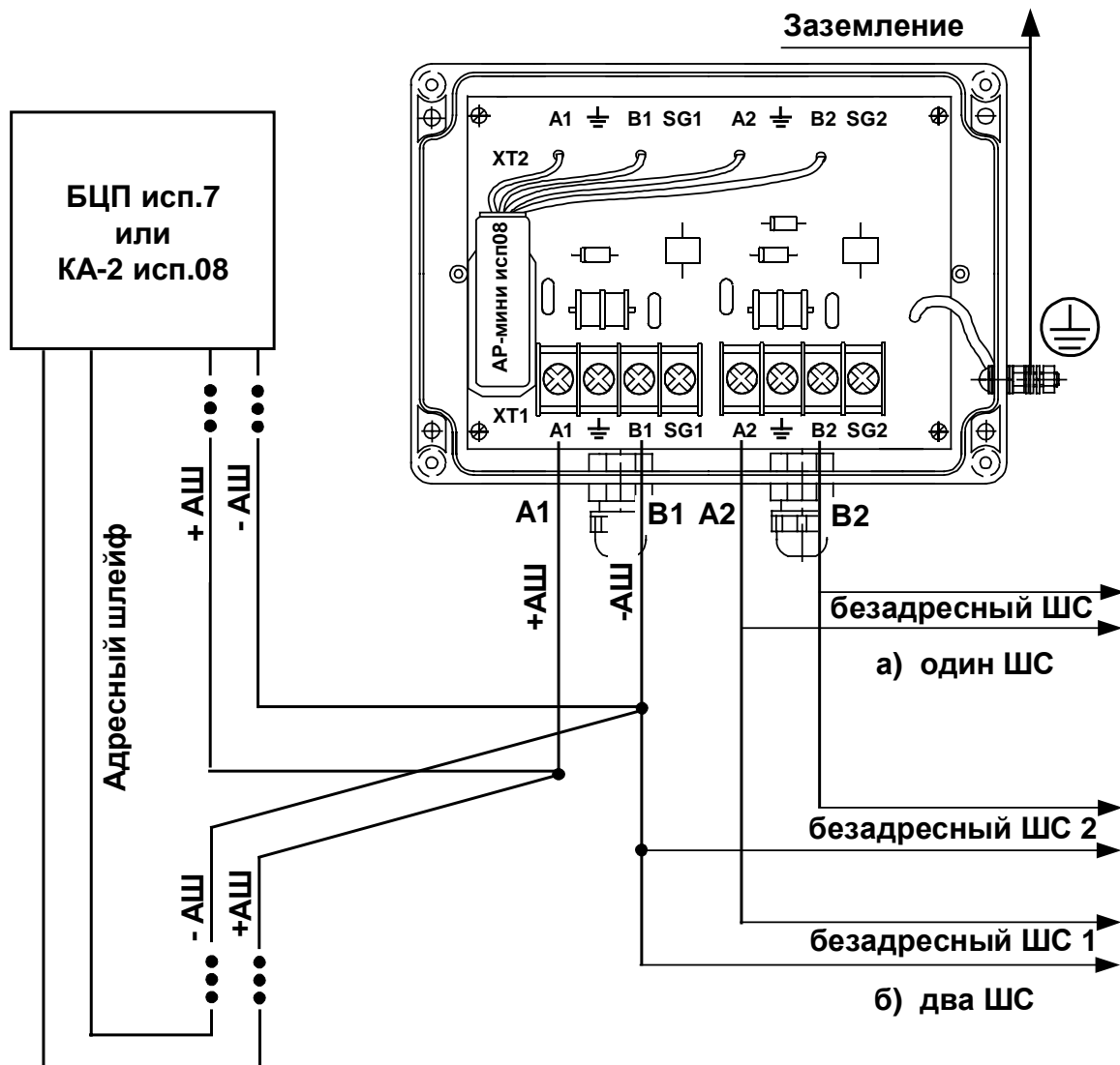
Рис. 12 Подключение Армини-П исп.08 а) один ШС; б) два ШС
