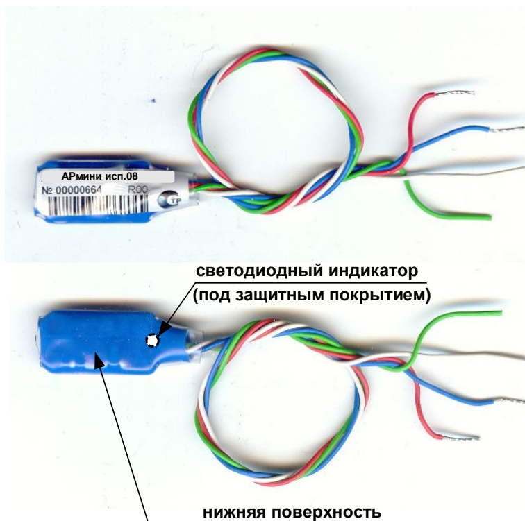
Рис. 1 Внешний вид АРмини исп.08
