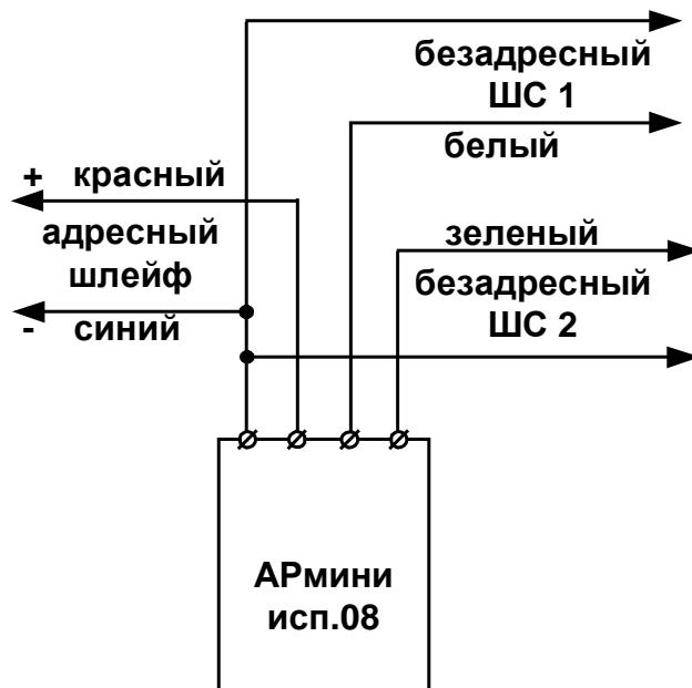
Рис. 3 Подключение устройства с двумя ШС
