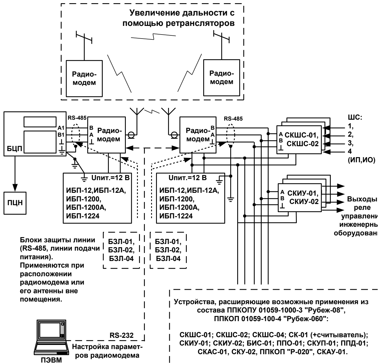
Рис. 1 Состав радиоканальной системы
