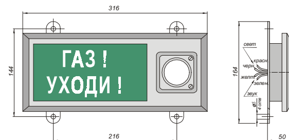
Оповещатель светозвуковой «Гамма-01 ОС3».
