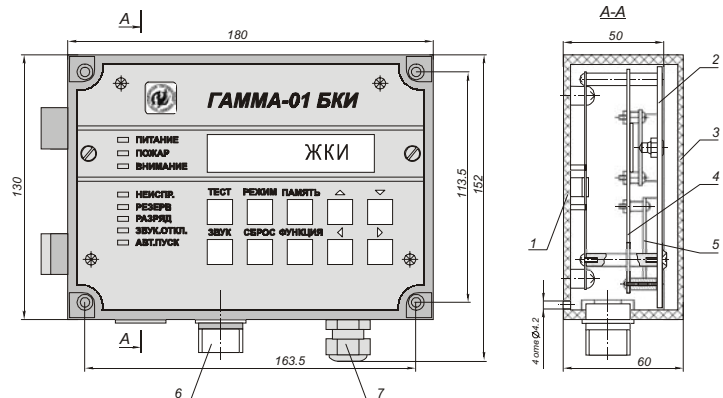
Блок клавиатуры и индикации «Гамма-01 БКИ»: 1 - корпус; 2 - панель; 3 - крышка; 4 - плата; 5 - плата; 6 - вилка 2PM22Б10Ш1В1; 7 - гермоввод.
