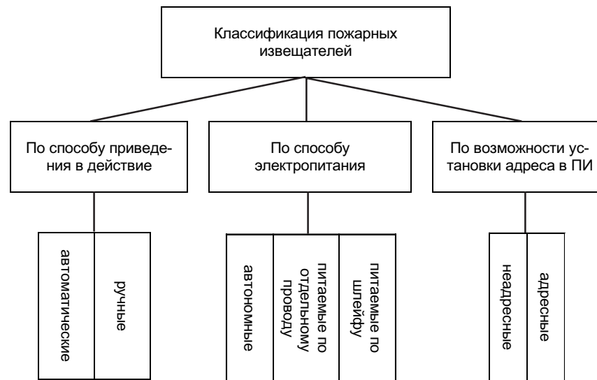
Рис. 2.5. Общая классификация пожарных извещателей.
