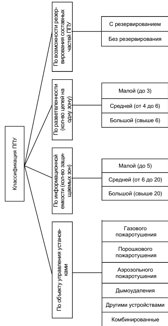
Рис. 2.4. Классификация приборов управления пожарных.
