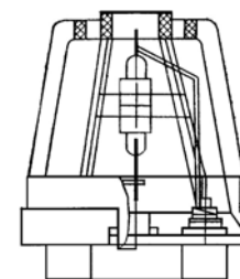
Рис. 1.4. Пожарный извещатель ИП105-2/1 (ИТМ)
