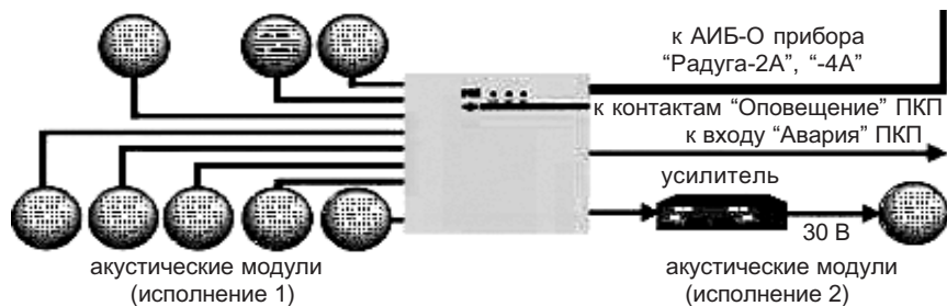
Схема подключения системы речевого оповещения «Орфей»
