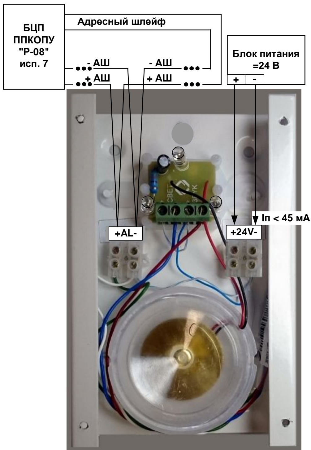
Рис. 3 Конструкция, подключение устройства
