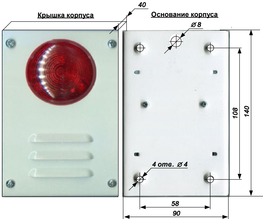
Рис. 2 Габаритные и присоединительные размеры
