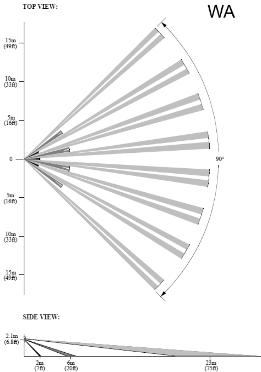
Рис. 4 Диаграмма зоны обнаружения при использовании линзы WA (вариант «О»)
