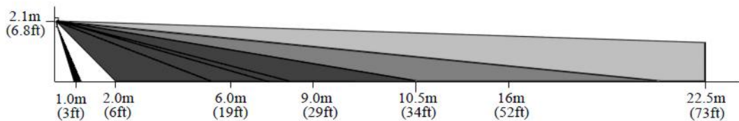
Рис. 5 Диаграмма зоны обнаружения СКАУ-01-Ш
