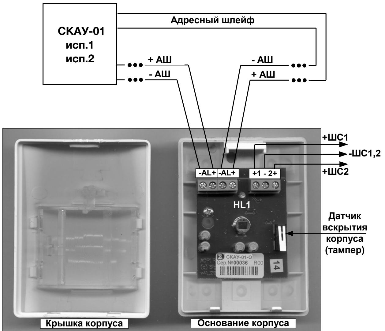
Рис. 2 Конструкция, подключение прибора
