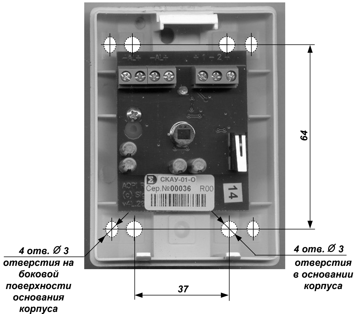
Рис. 3 Присоединительные размеры корпуса прибора
