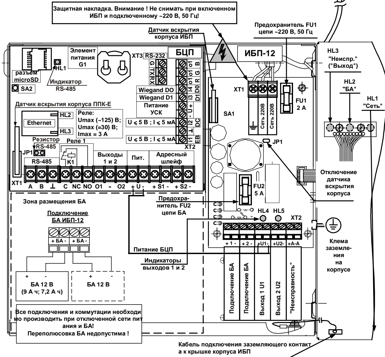
Рис. 10 Внешний вид БЦП исп. 7-1У
