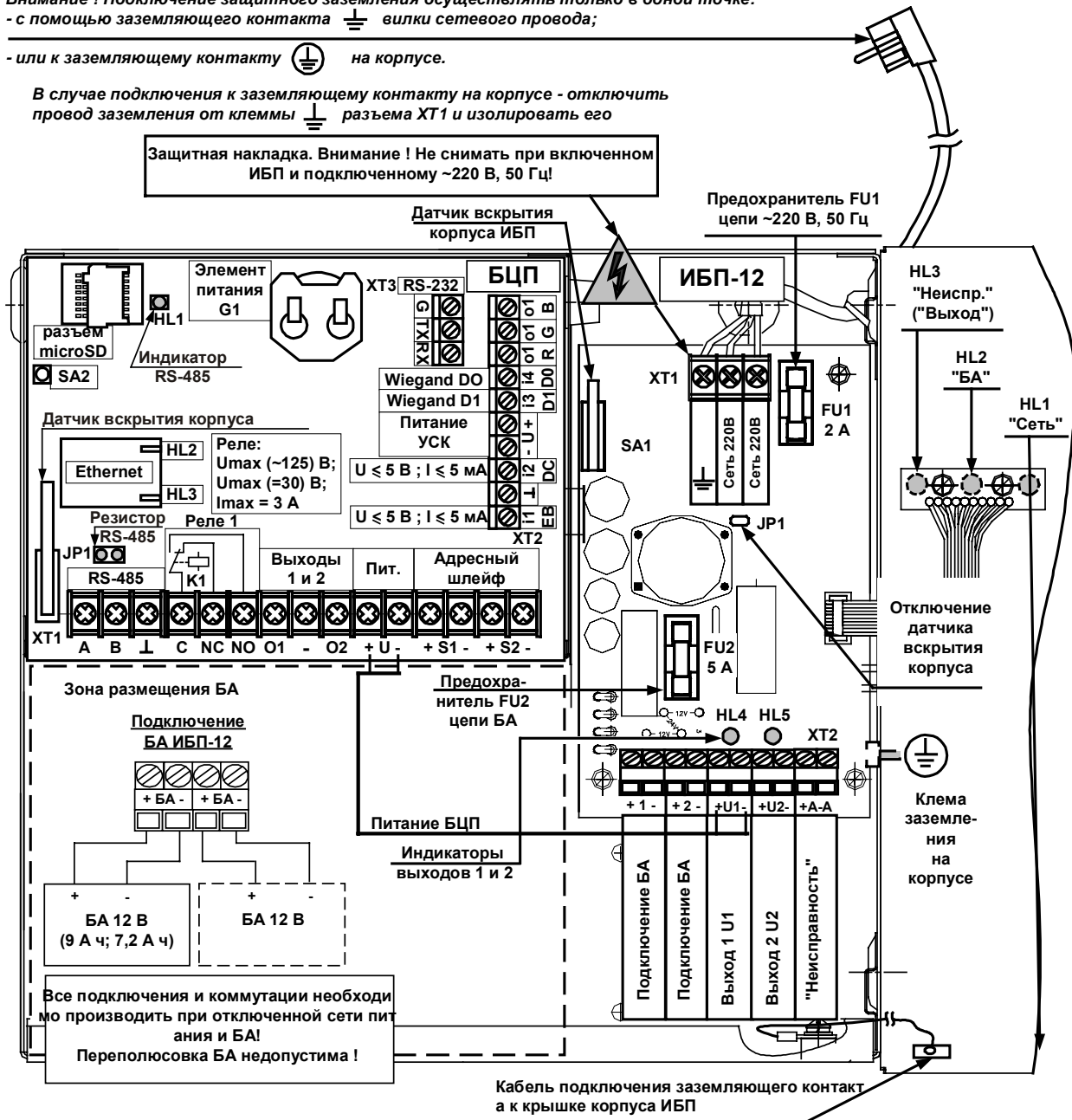
Рис. 9 Внешний вид БЦП исп. 7-1
