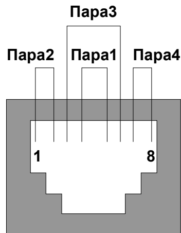
Рис. 6 Подключение ППК и ПЭВМ (Ethernet)
