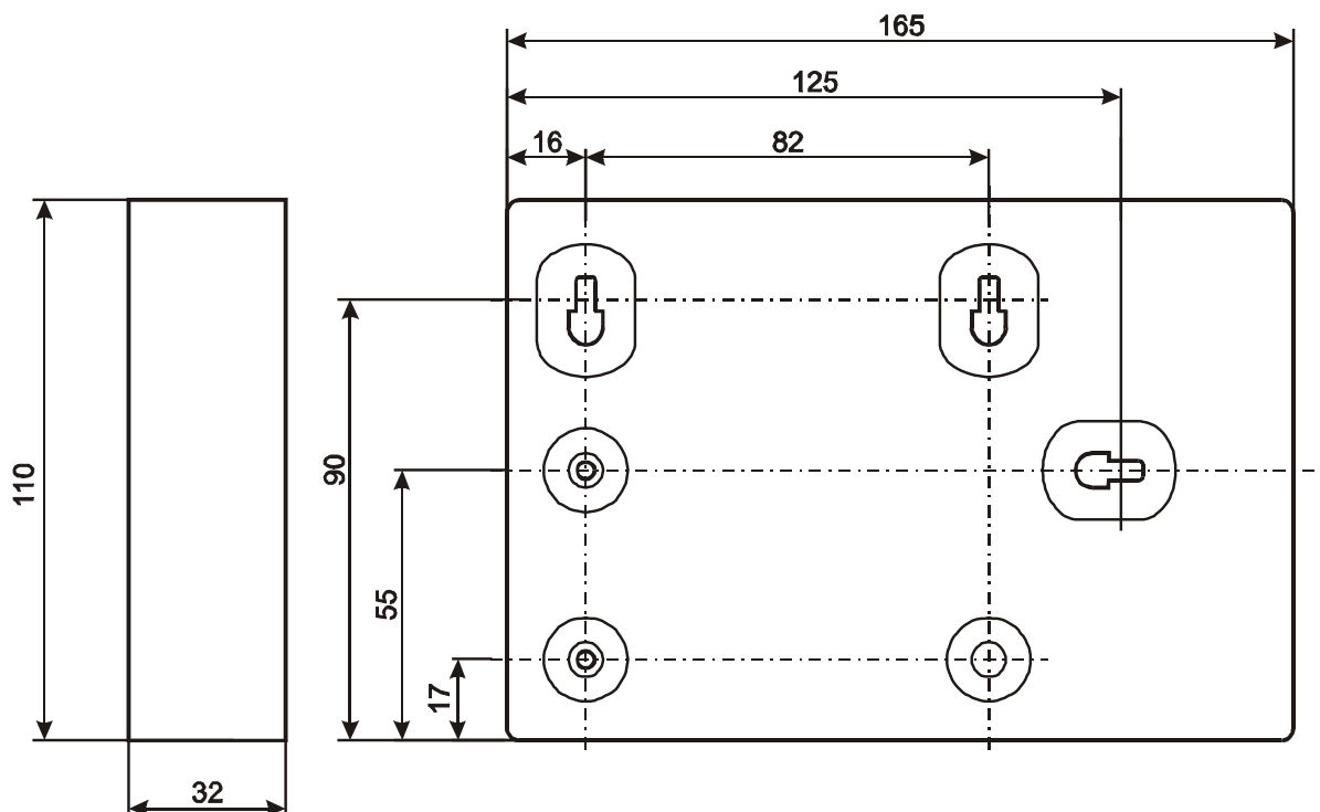
Рис. 2 Габаритные и присоединительные размеры корпуса ТИ
