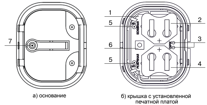
Рисунок 1 – Конструкция извещателя
