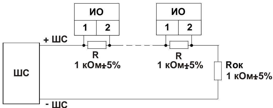
Рис. Схема 2 ИО с нормально-замкнутыми контактами (с контролем обрыва ШС, не более 3-х ИО)
