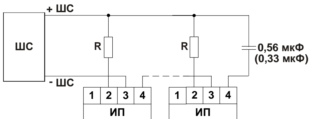
Рис. Схема 3 ИП с нормально-разомкнутыми контактами (типа ИП-212М и т.п.). R см. Табл. 5
