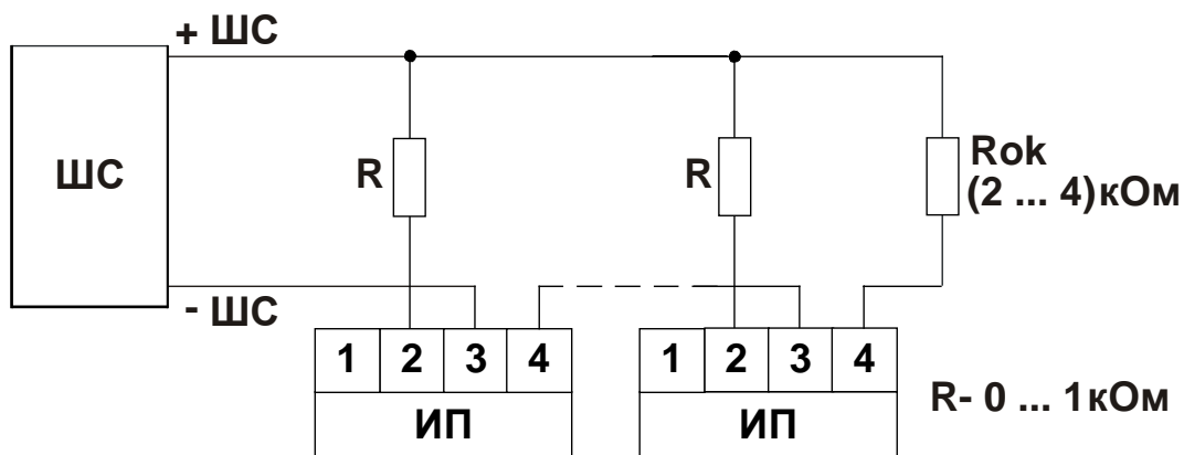
Рис. Схема 4 ИП Т7[Н.Р.] с нормально-разомкнутыми контактами, токопотребляющие (типа ИП-212М и т.п.). R см. Табл. 5
