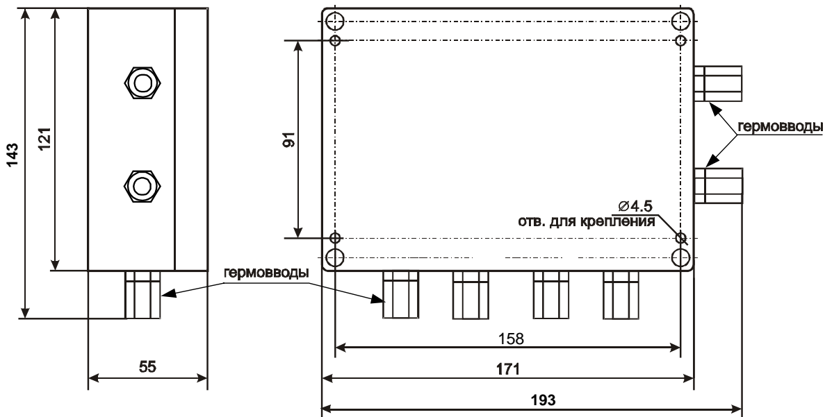
Рис. 3 Габаритные и присоединительные размеры (исп. IP65)
