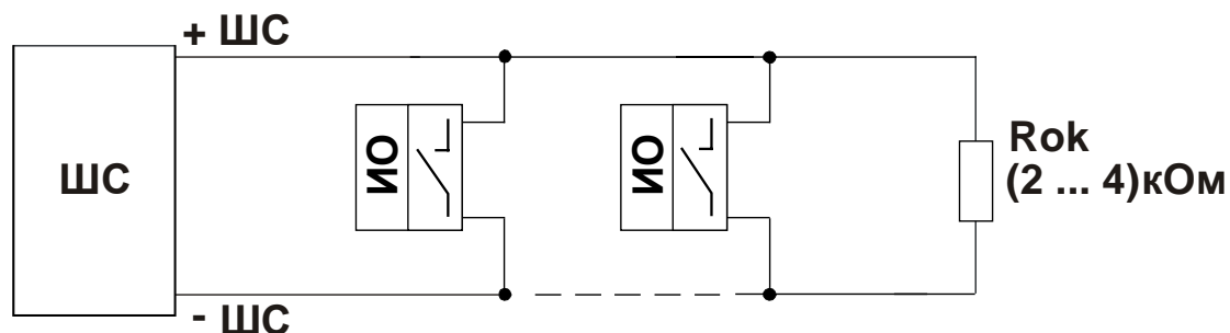
Рис. Схема 6 ИО с нормально-разомкнутыми контактами
