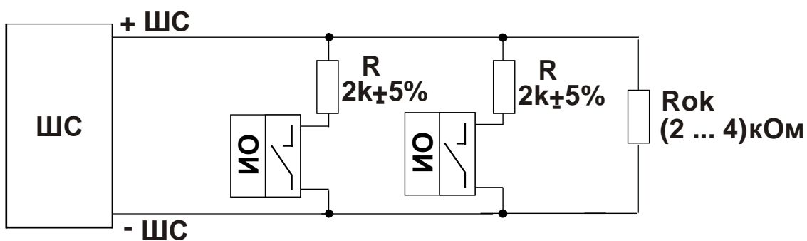
Рис. Схема 5 ИО с нормально-разомкнутыми контактами (Тип 7, не более 2-х извещателей)
