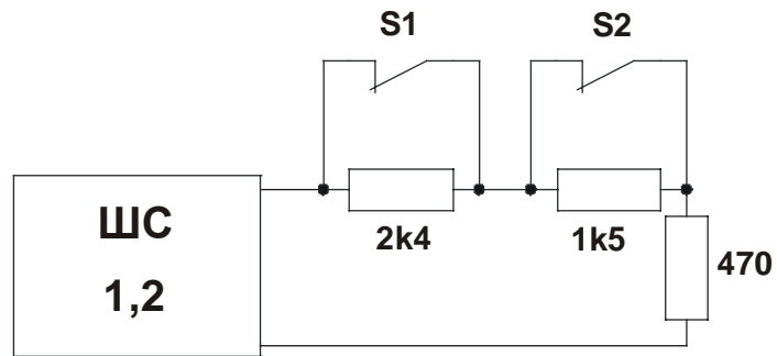
Схема 1 Последовательное подключение 2-х извещателей с НЗ контактами.
