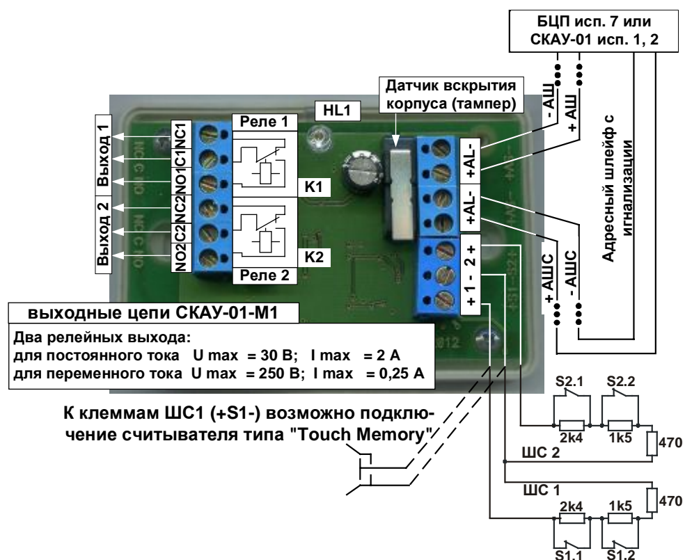
Рис. 2 Подключение СКАУ-01-М1
