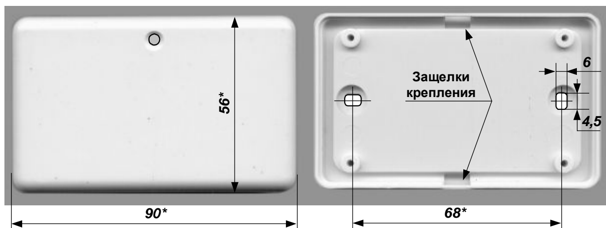
Рис. 3 Габаритные и присоединительные размеры корпуса SKAU-01-M1
