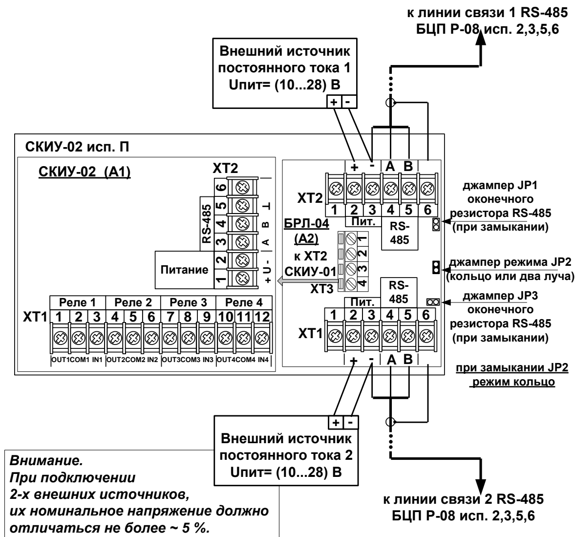
Рис. 2 Применение (подключение) СКИУ-02 П в режиме кольца линий связи RS-485
