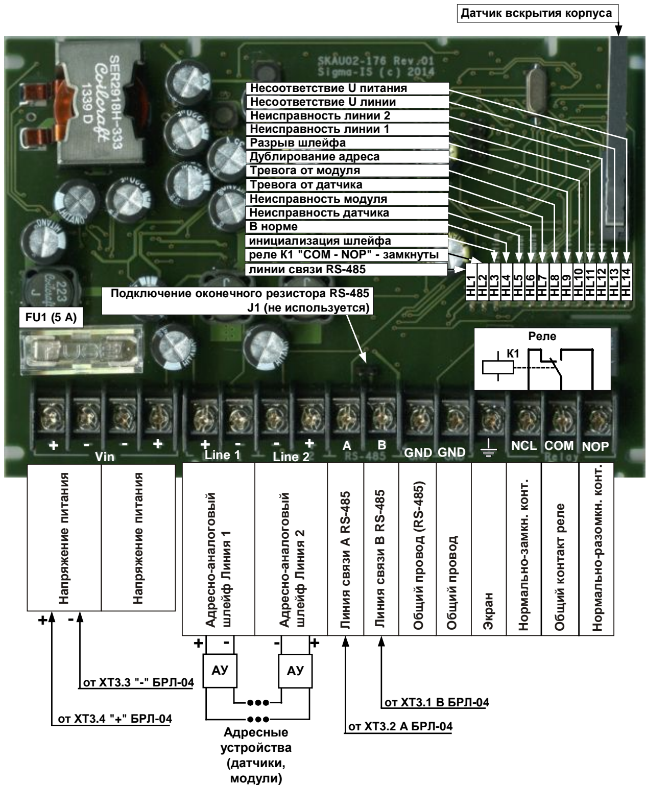
Рис. 4 Внешний вид модуля SKAU-02(A1) . Подключение.
