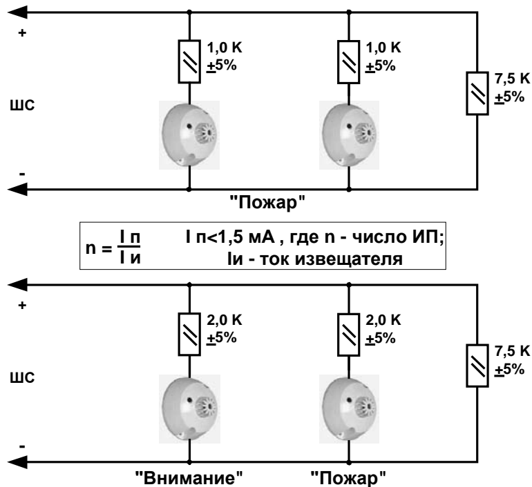
Рис. 12 Подключение извещателя пожарного типа ИП101-1А, ИП212-73("ПРОФИ-О") с базой V401 (с формированием извещений «Пожар» и «Внимание» - «Пожар»)
