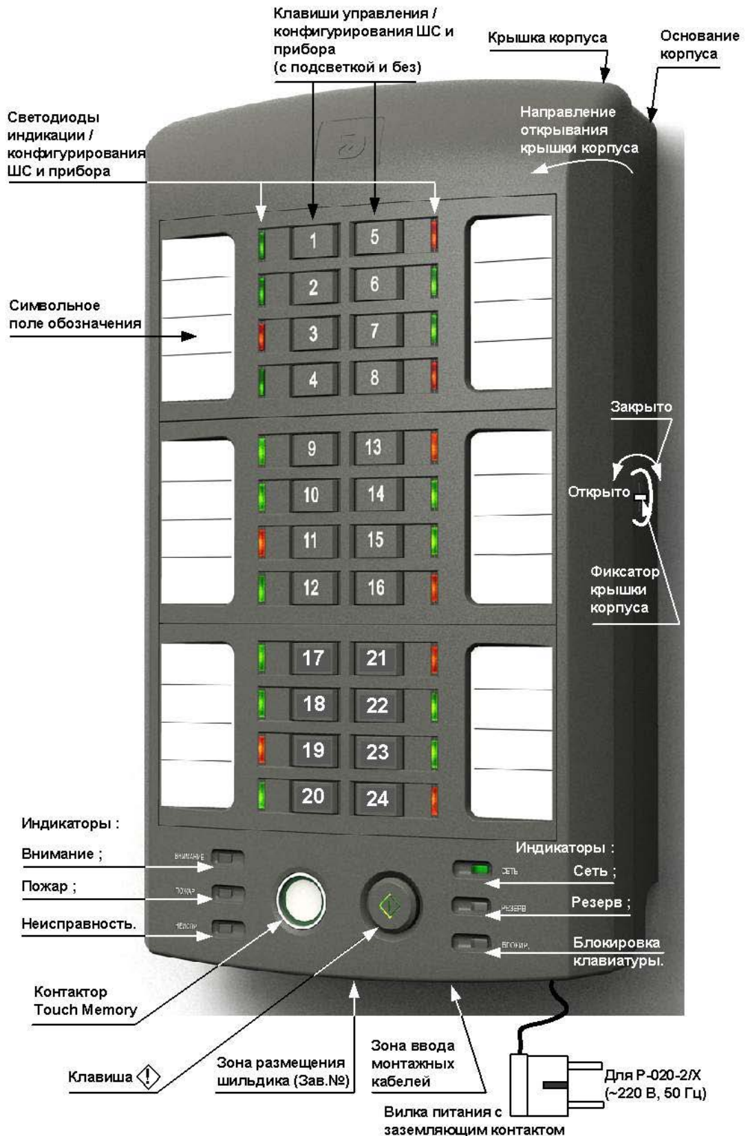
Рис. 1 Внешний вид прибора
