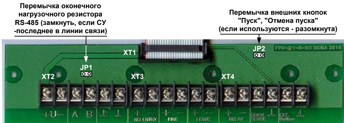
Рис. 3 Расположение элементов на плате подключения
