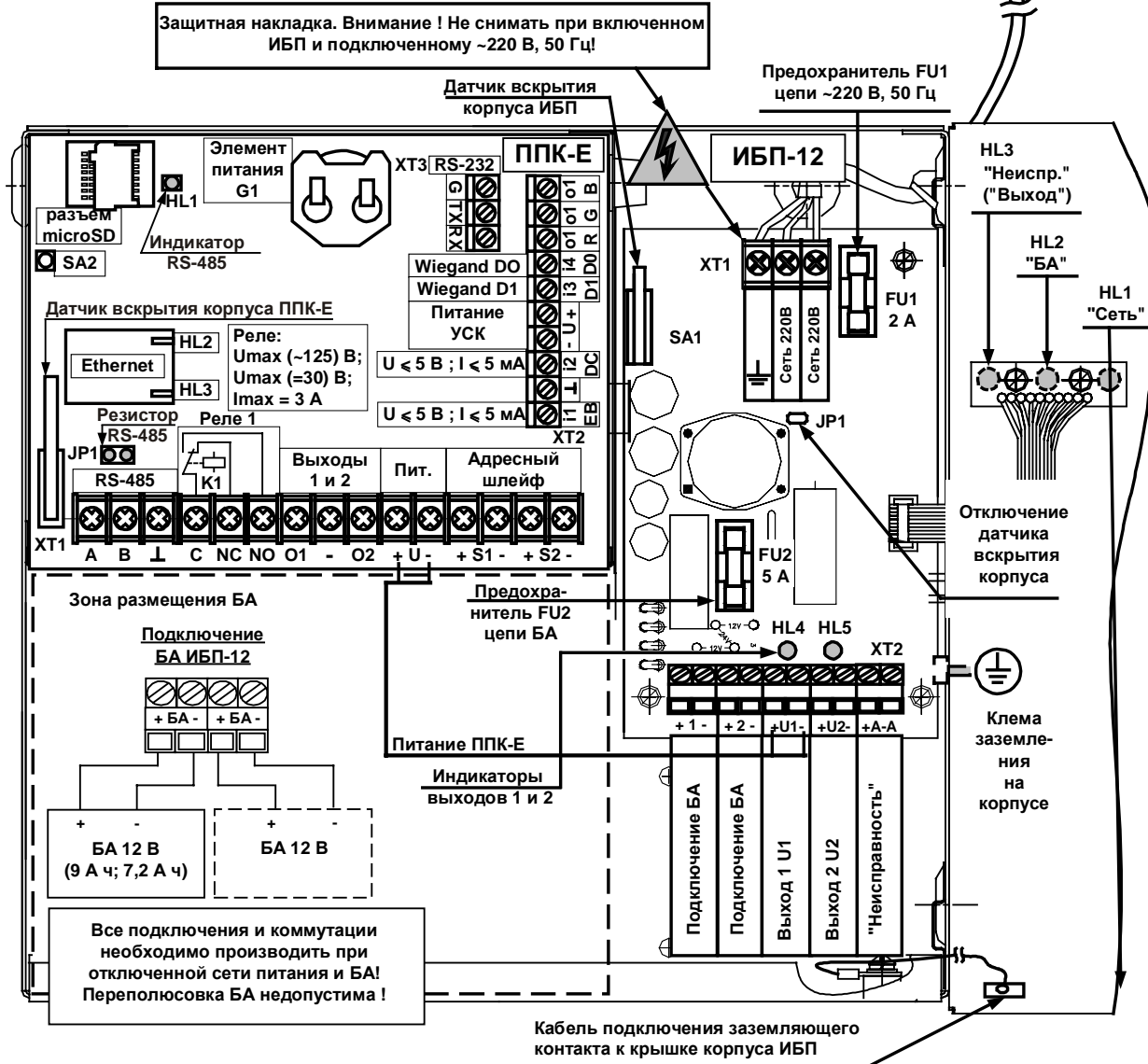
Рис. 11 Внешний вид ППК-Е (исп. 1)
