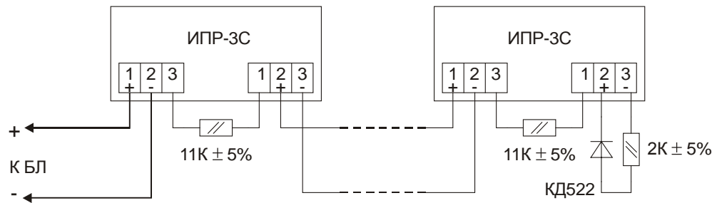
Рис. 23 Схема включения ИПР-3С
