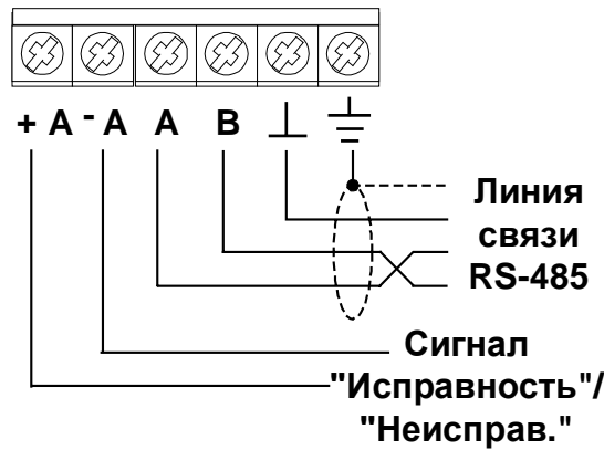
Рис. 5 Подключение линий связи: RS-485 и сигнала "Исправность"/"Неисправ." ИБП
