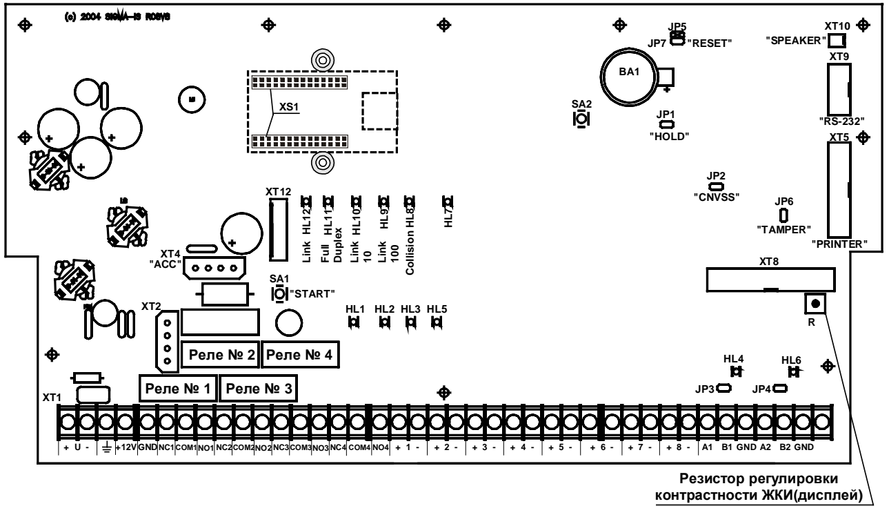
Рис. 31 Плата БЦП исп. 2,3
