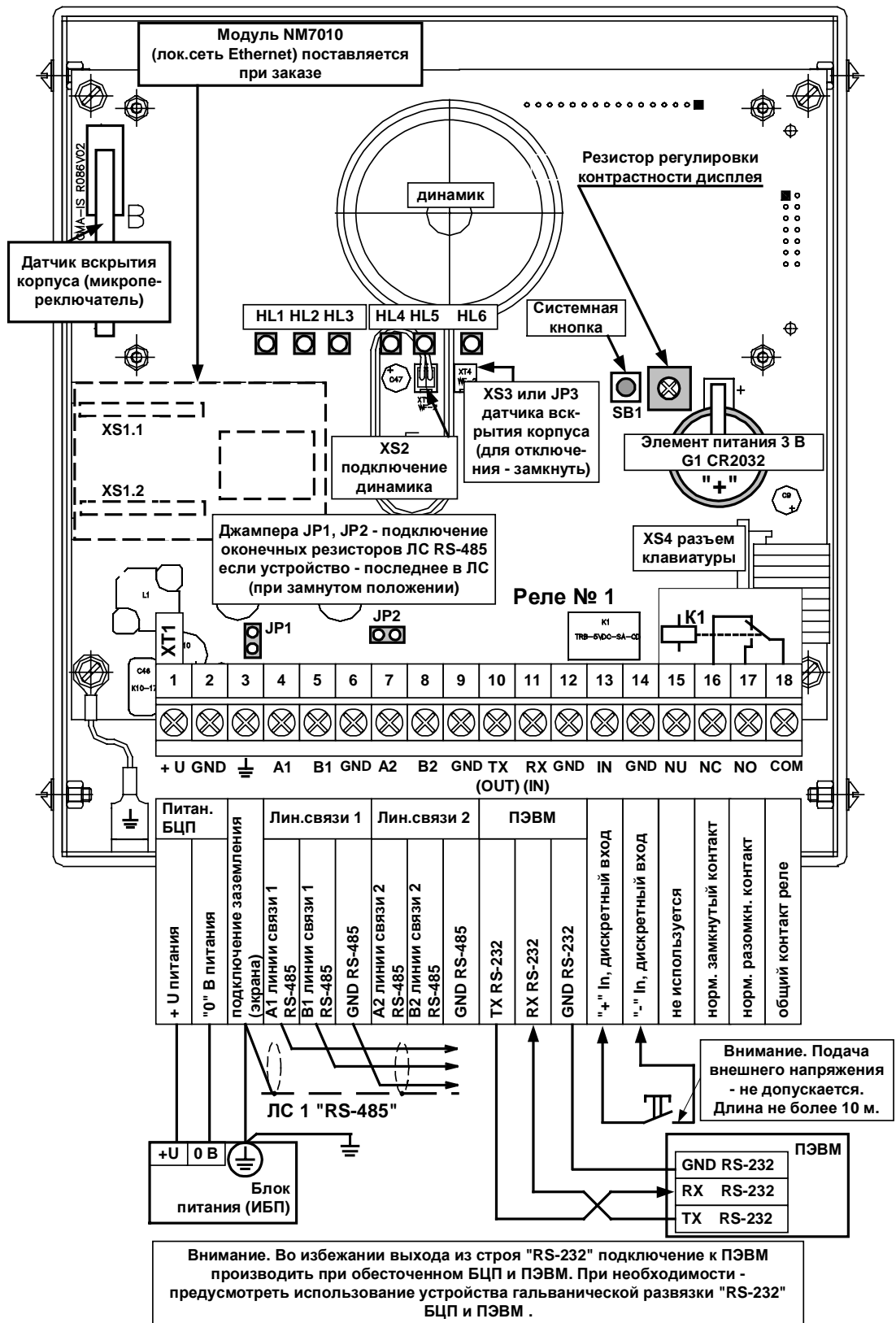
Рис. 40 Расположение элементов и подключение БЦП исп. 6
