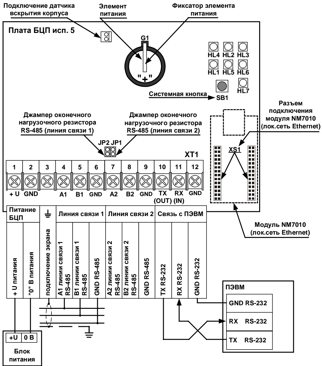
Рис. 37 БЦП исполнения 5
