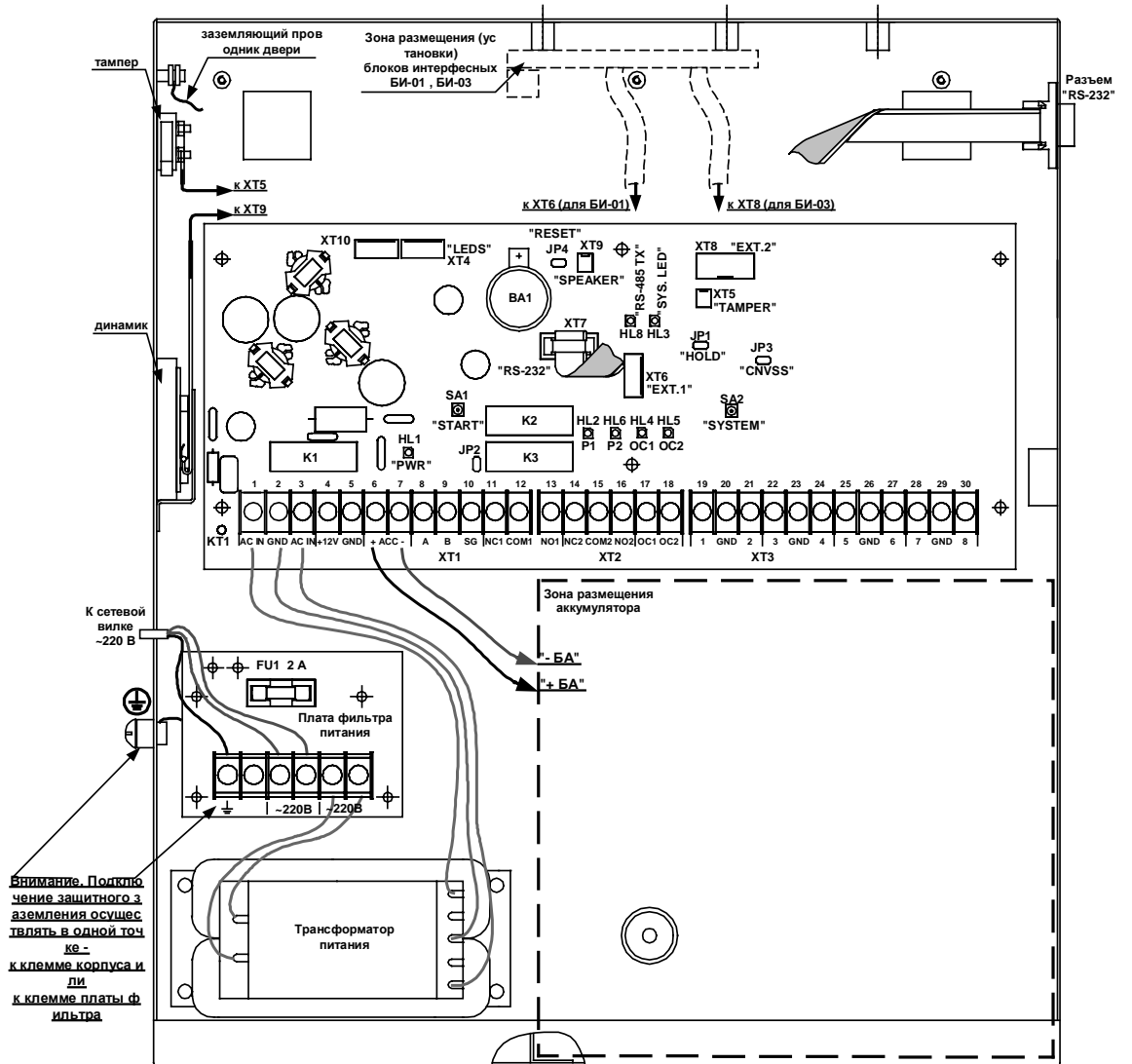
Рис. 34 Расположение элементов БЦП исп.4
