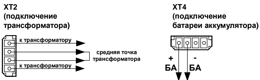
Рис. 30 Разъемы ХТ2 и ХТ4 исп. 3
