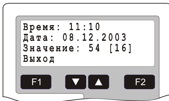
Рис. 31 Журнал СКАУ-01
