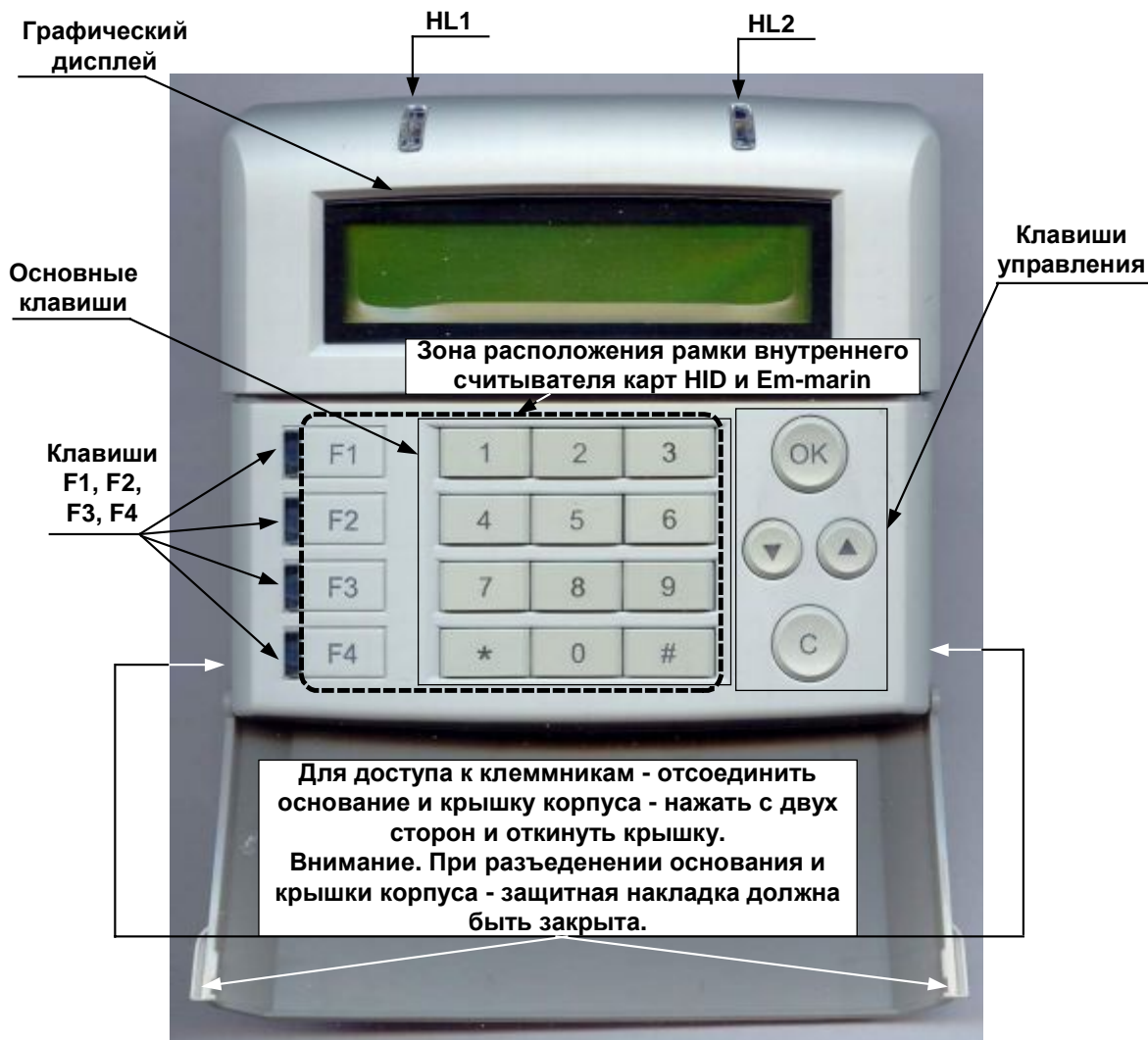
Рис. 2 Внешний вид ПУО (с откинутой накладкой)
