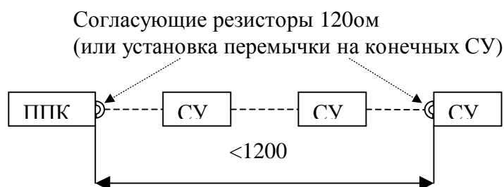
Рис. 5 Подключение сетевых устройств на линию RS-485.
