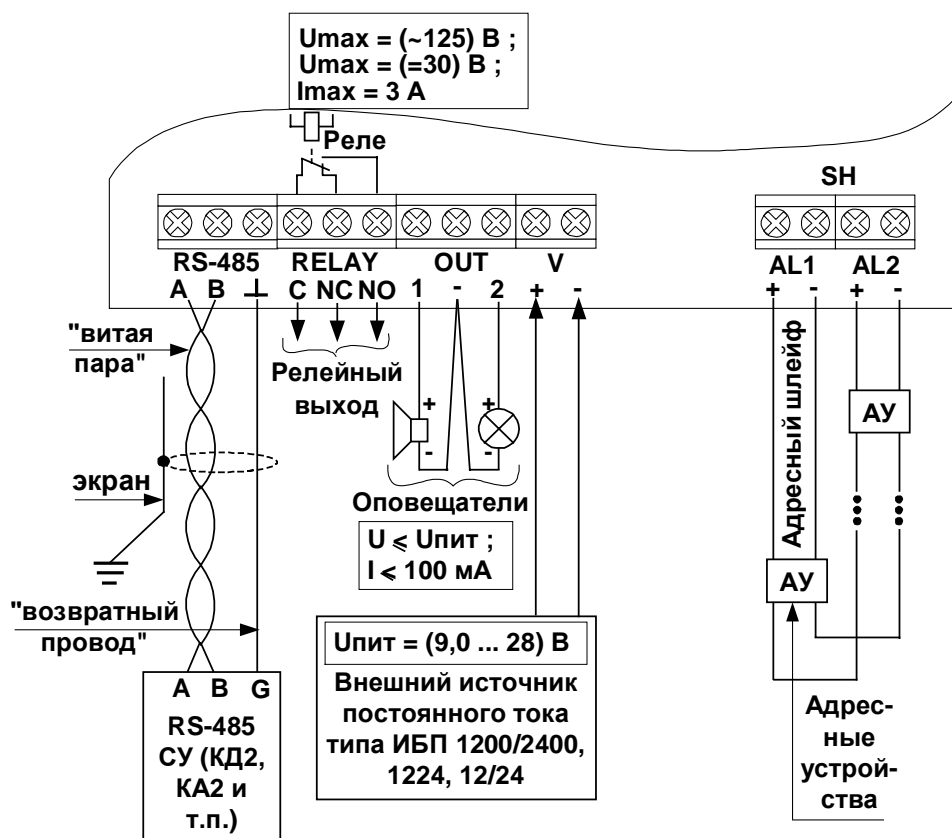
б) Вариант ППК. ППК-М без выходов 1 и 2 ПЧН (ППК – с зав. № 240 и ППК-М – с зав. № 290)
