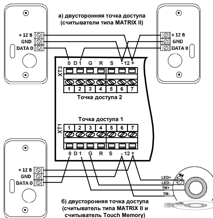
Рис. 9 Подключение считывателей при двусторонней ТД
