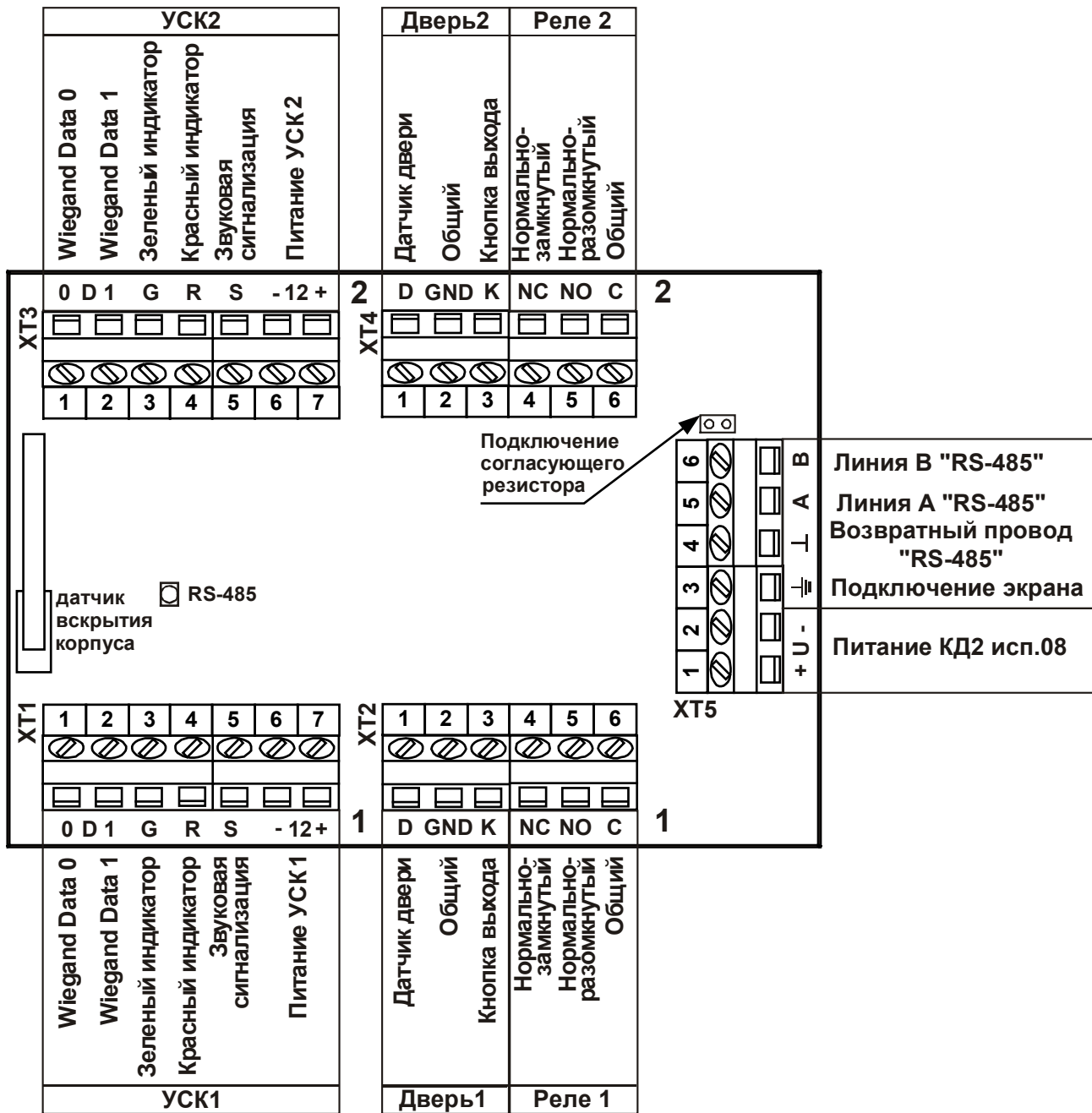
Рис. 6 Клеммы подключения КД2
