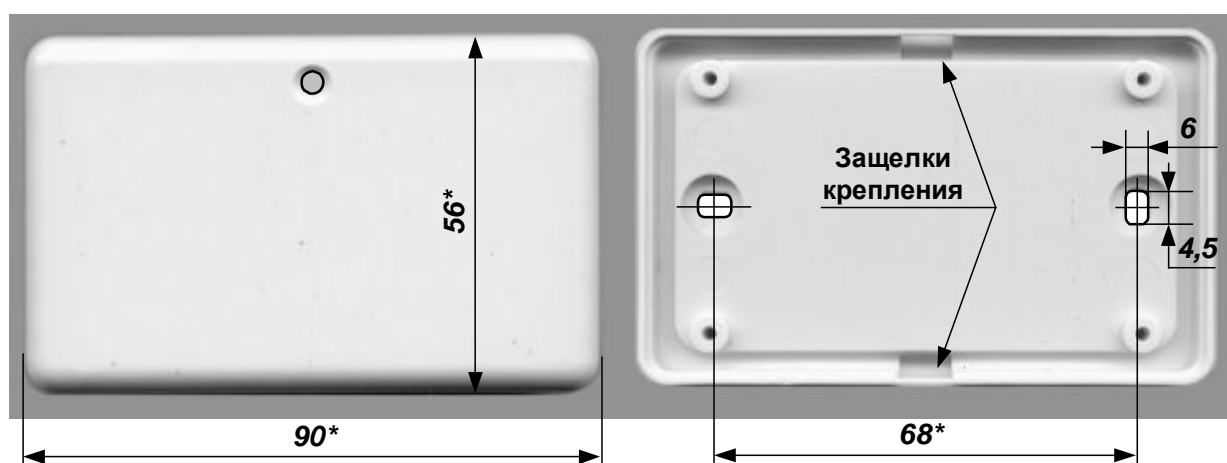
Рис. 2 Внешний вид, габаритные и присоединительные размеры (исполнение IP20)
