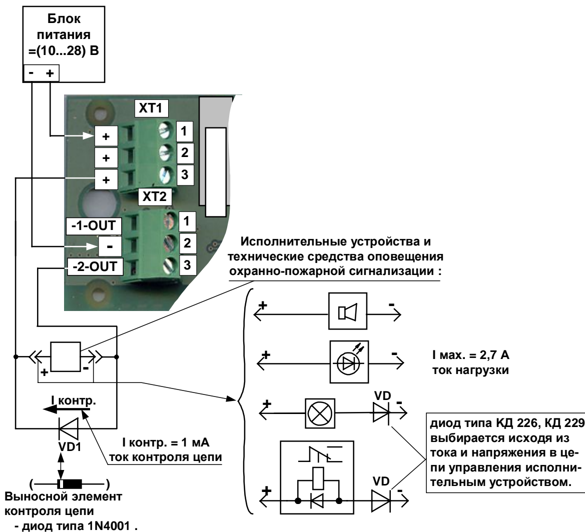
Рис. 3 Подключение исполнительного устройства к выводу 2 (в скобках показана маркировка диода 1N4001 при подключении)
