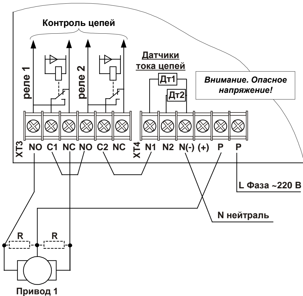
Рис. 7 Подключение 1-го реверсивного привода переменного тока типа Белимо с возможностью отключения напряжения
