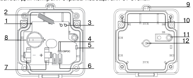
а) основание с установленной печатной платой
