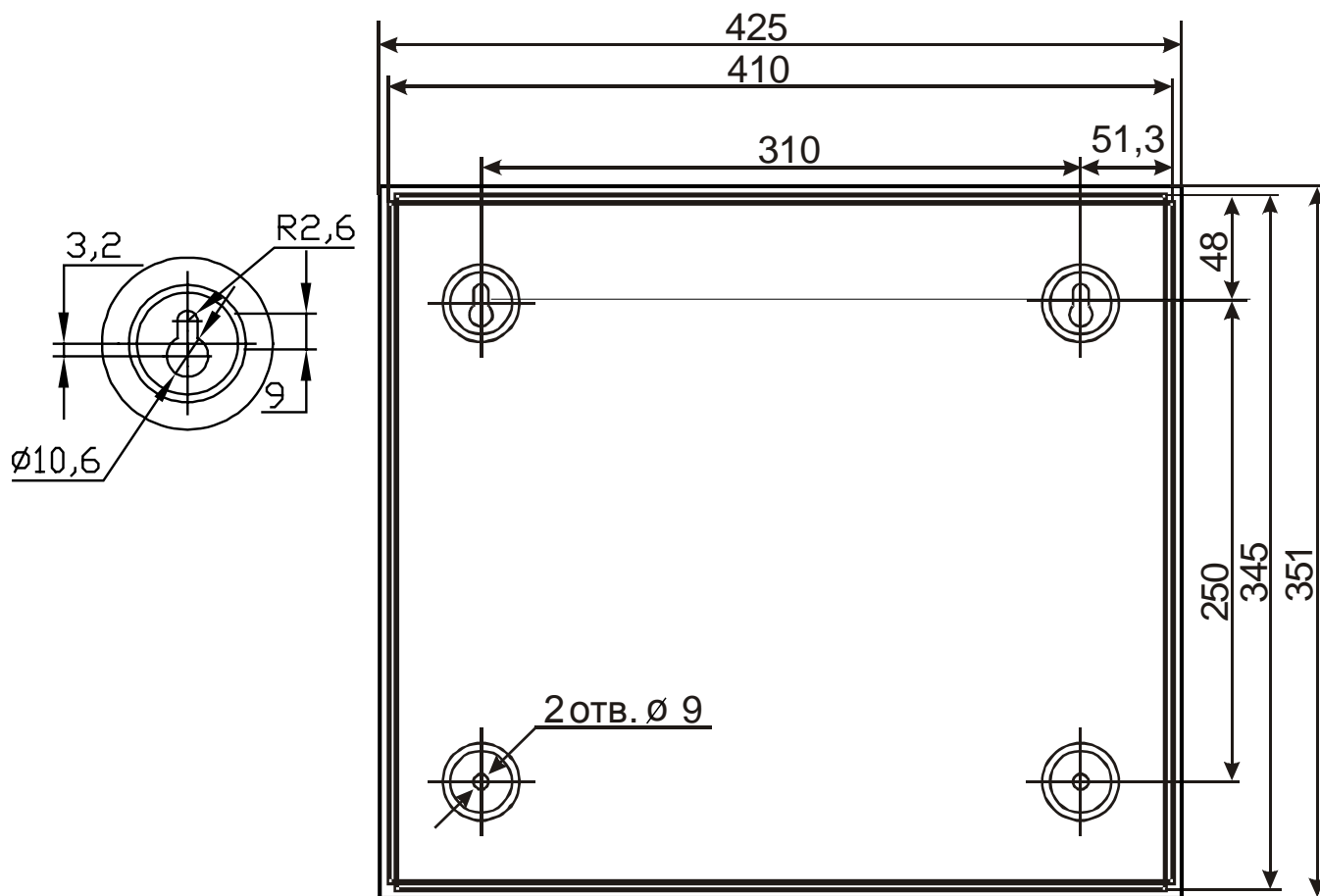
Рис. 10 Присоединительные размеры ИБП 1200/2400
