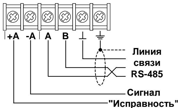
Рис. 6 Подключение линий связи: RS-485 и сигнала "Исправность"
