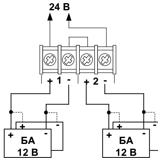
Рис. 8 Подключение аккумуляторных батарей в ИБП2400
