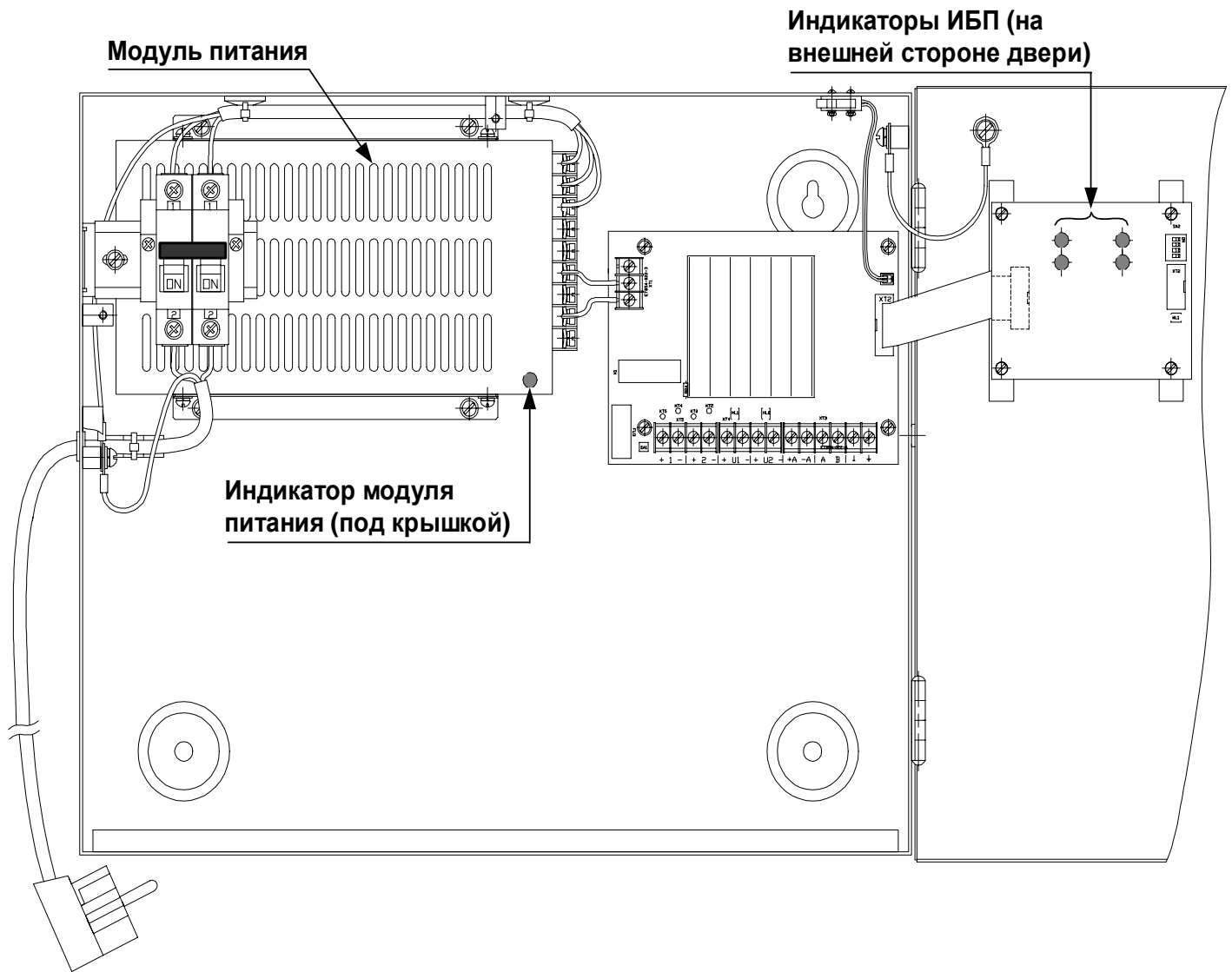
Рис. 3 Внешний вид ИБП без фальшпанели
