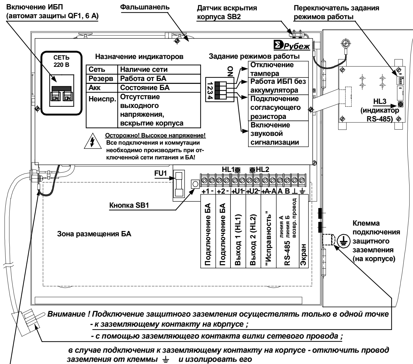
Рис. 2 Внешний вид ИБП с открытой дверью
