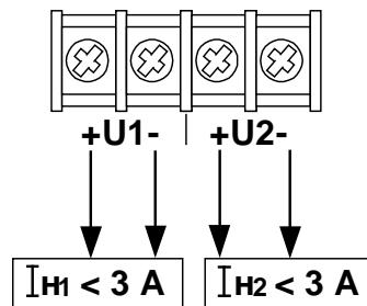
Рис. 4 Схема подключения нагрузки ( I_{n1} < 3A ; I_{n2} < 3A )
