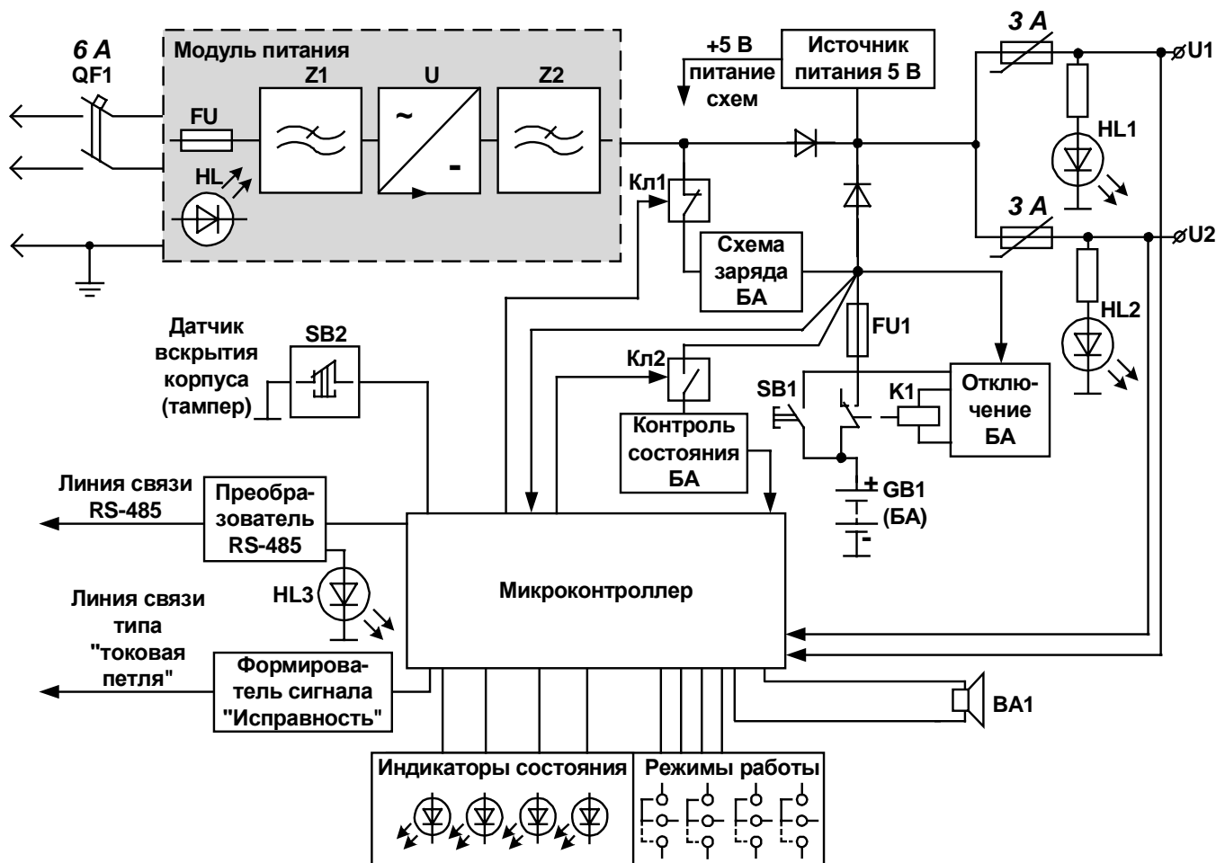
Рис. 1 Электрическая функциональная схема ИБП 1200/2400
