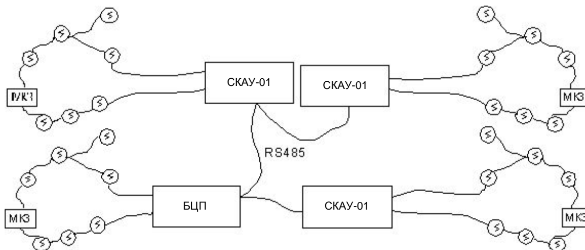
Рис. 7 Подключение адресных устройств при помощи SKAY-01 исп.1 и 2
