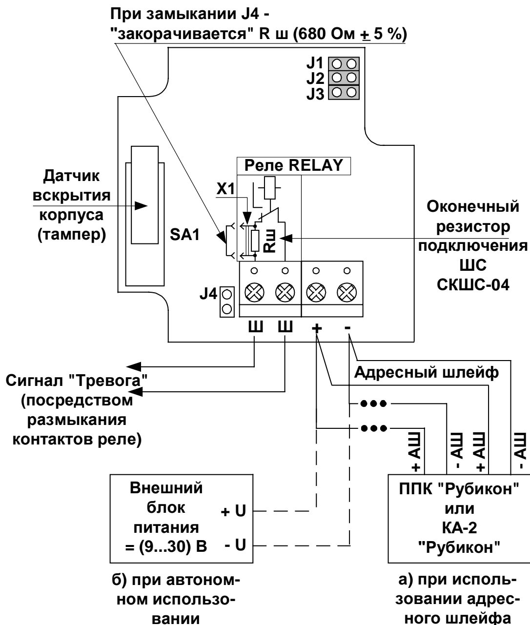
Рис. 2 Плата, подключение АВИ: а) при использовании адресного шлейфа (ППК или КА-2 “Рубикон”) ; б) при автономном использовании.
