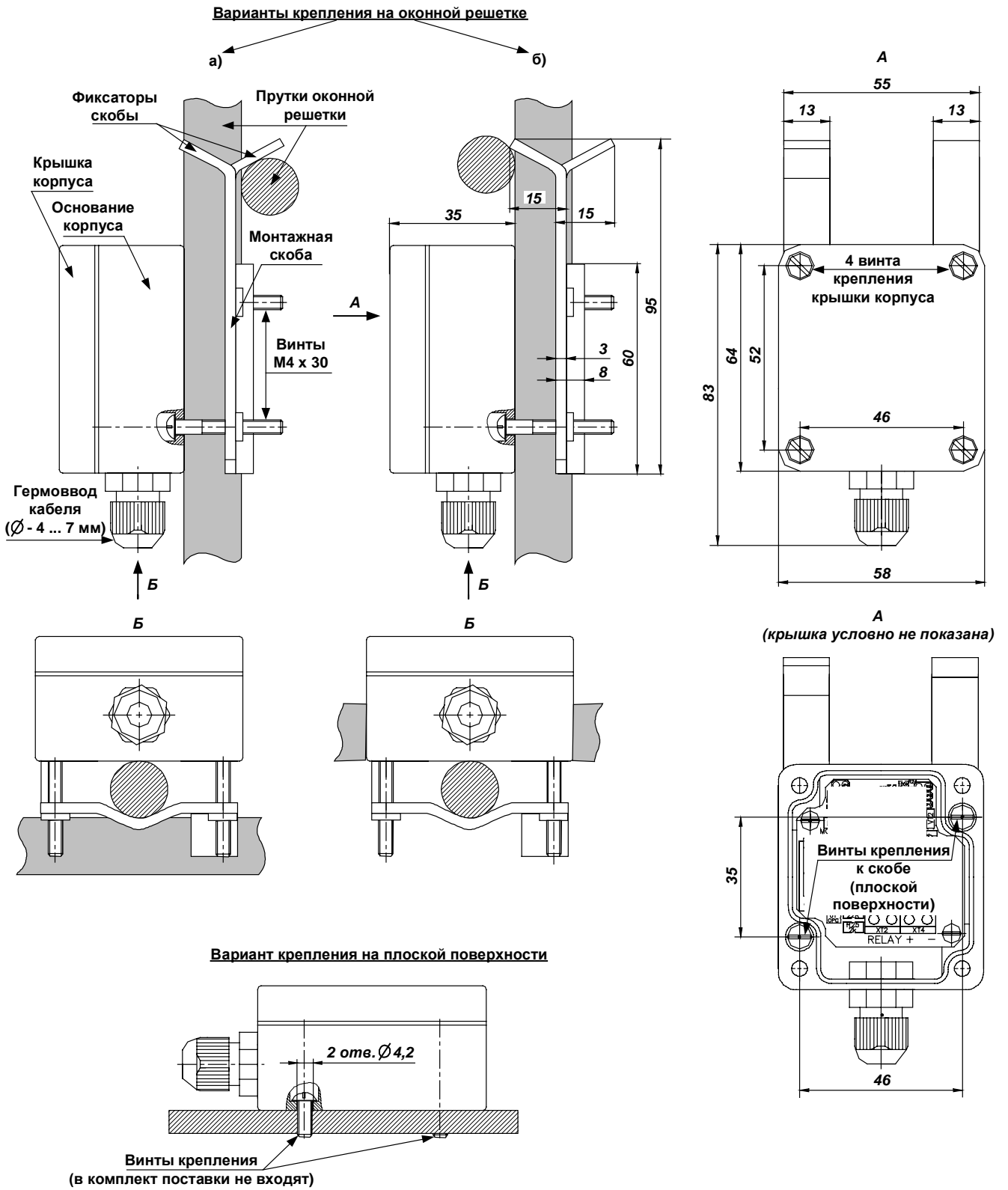
Рис. 1 Внешний вид, варианты крепления, габаритные и установочные размеры.
