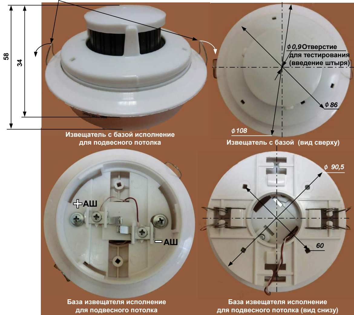
Рис. 2 АТИ (блок извещателя, база). Габаритные и присоединительные размеры.
