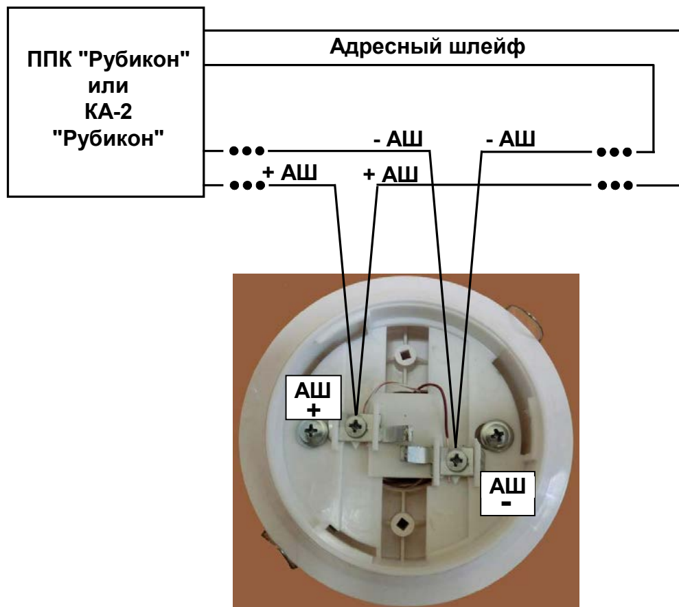
Рис. 3 Подключение АТИ
