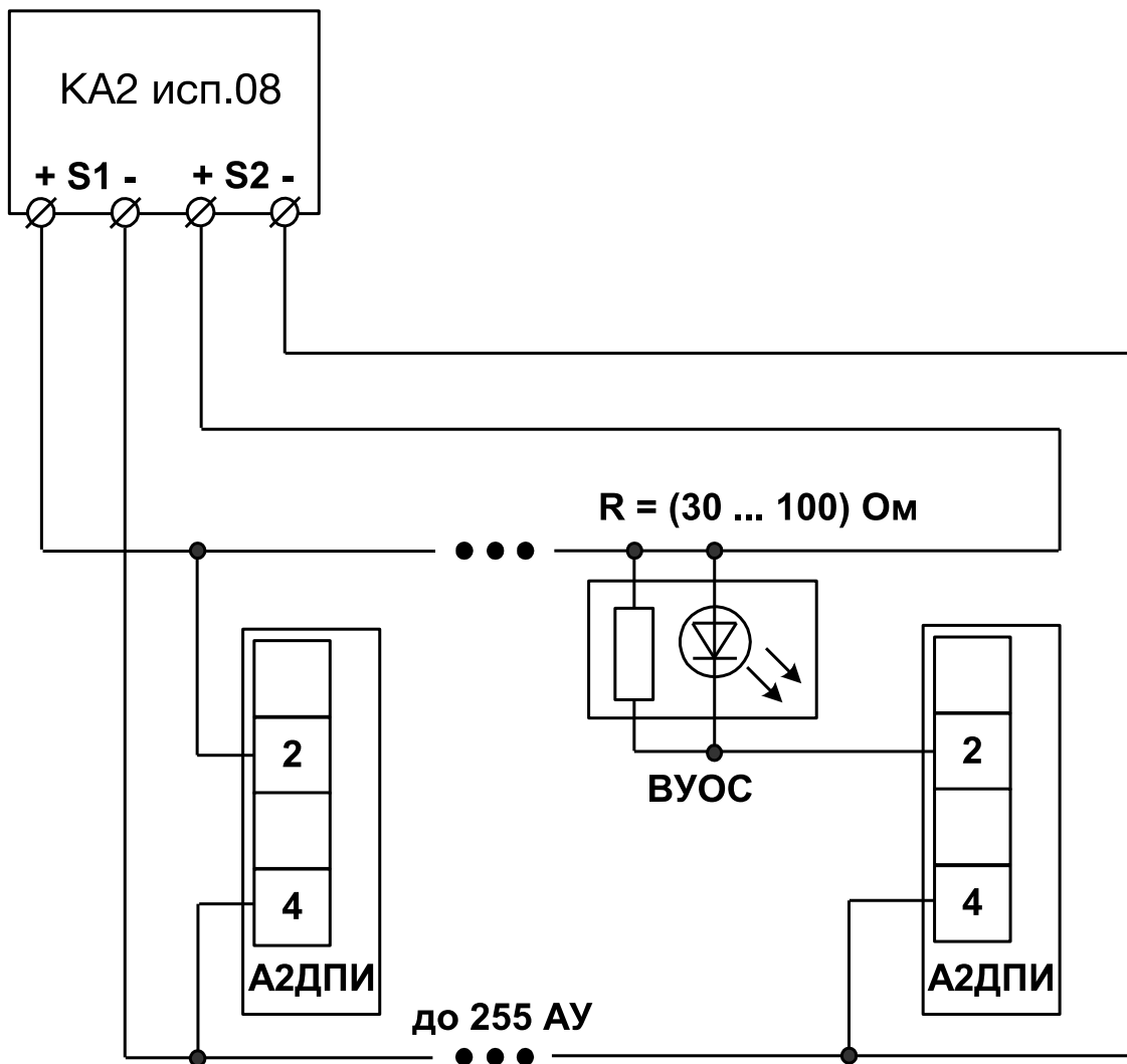
Рис. 4 Подключение А2ДПИ в АШ КА2 исп.08
