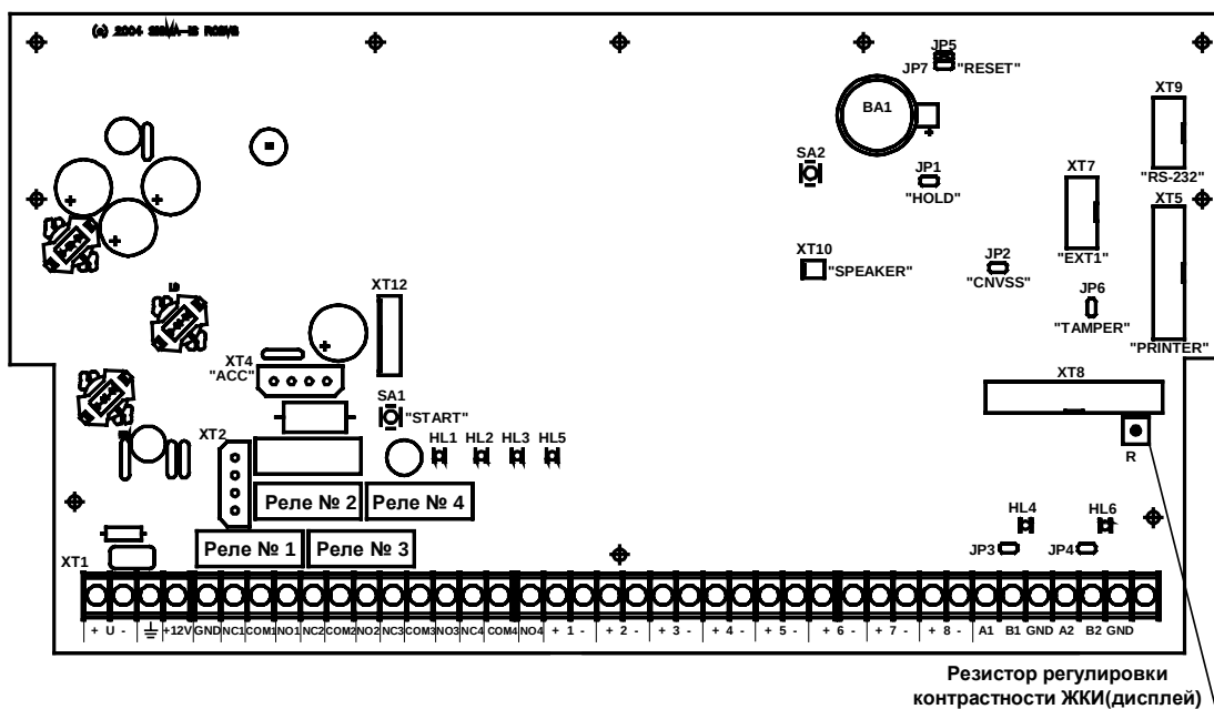
Рис. 31 Плата БЦП исп. 1,2,3
