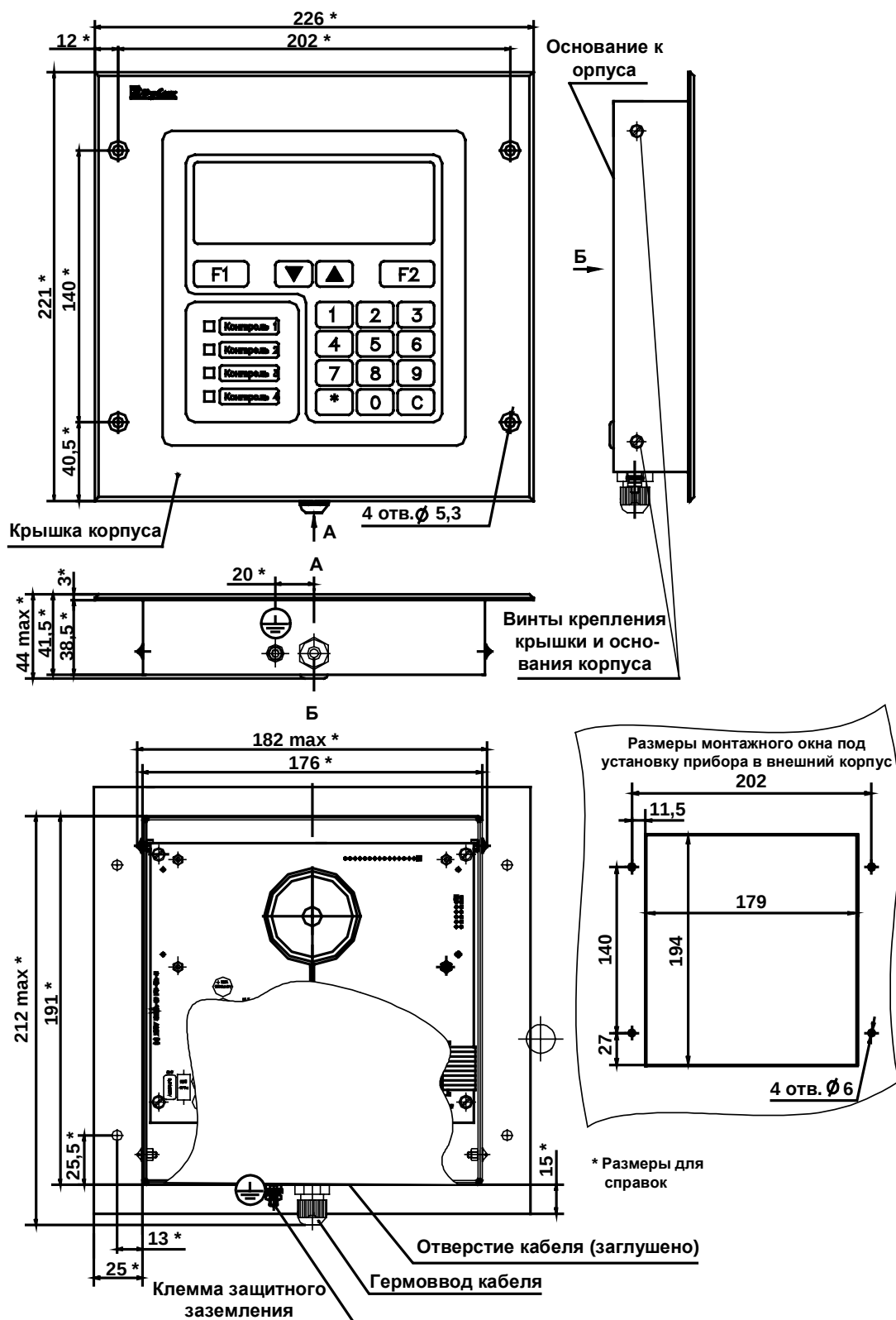
Рис. 42 Габаритные и присоединительные размеры БЦП исп. 6В и исп. 6ВК (IP54, врезной вариант)
