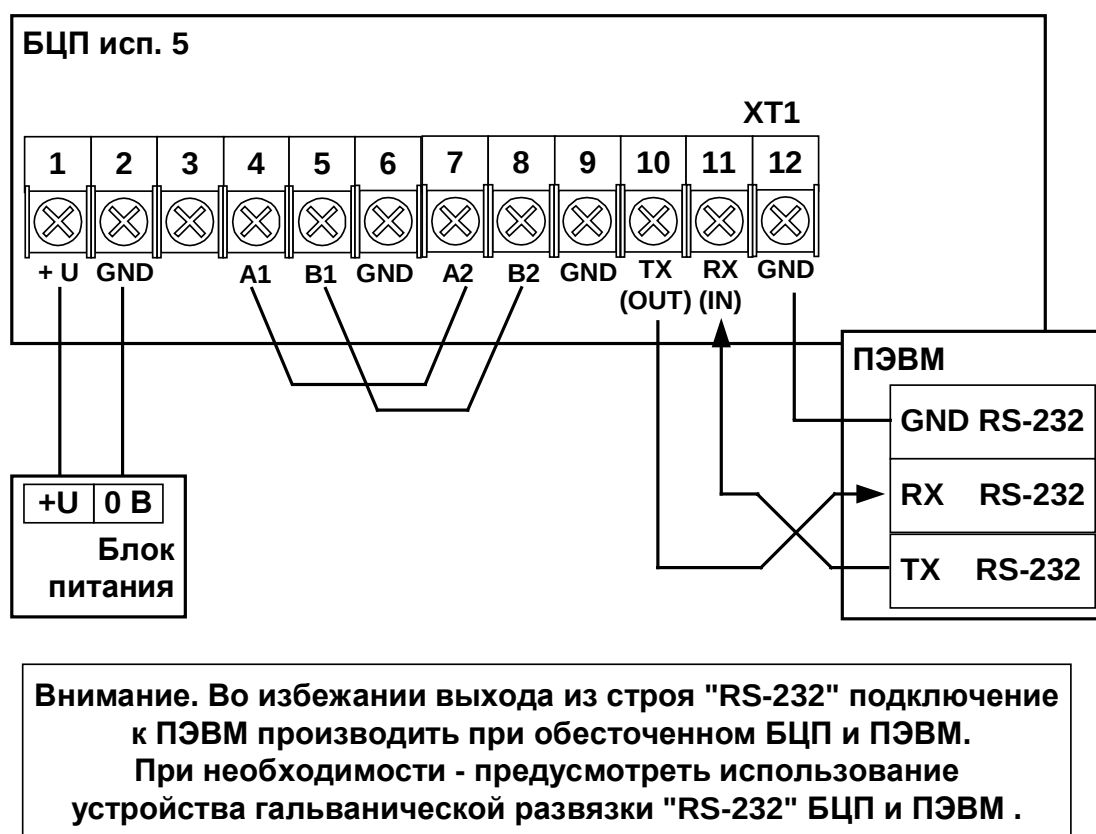
Рис. 43 Схема проверки БЦП исп. 5
