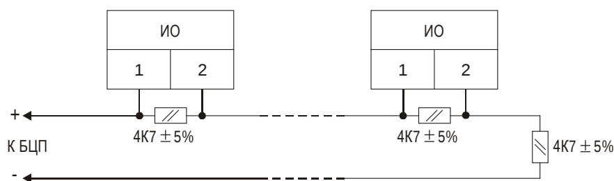
Рис. 19 Подключение ШС для типа 2
