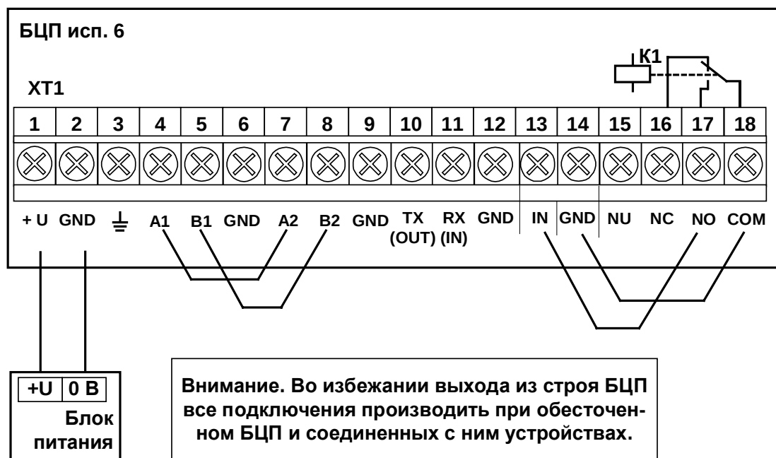
Рис. 44 Схема проверки БЦП исп. 6
