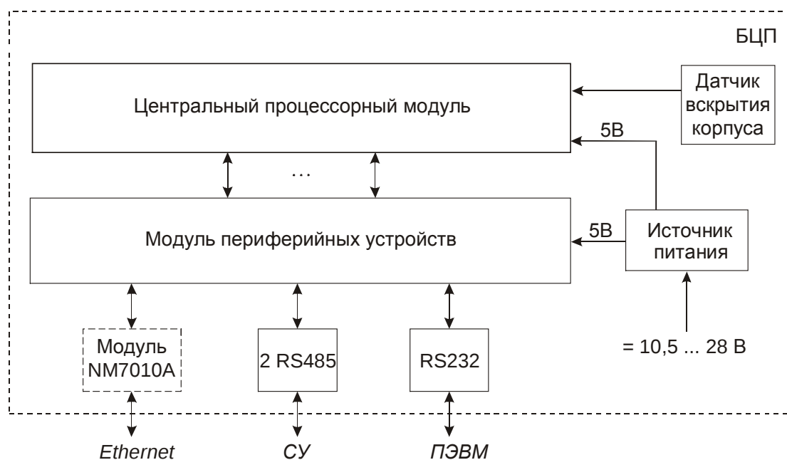
Рис. 5 Электрическая структурная схема БЦП Р-08 исп. 5
