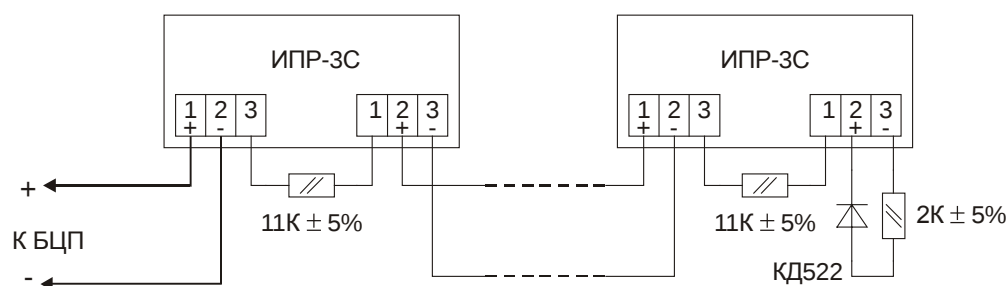
Рис. 27 Схема включения ИПР-ЗС
