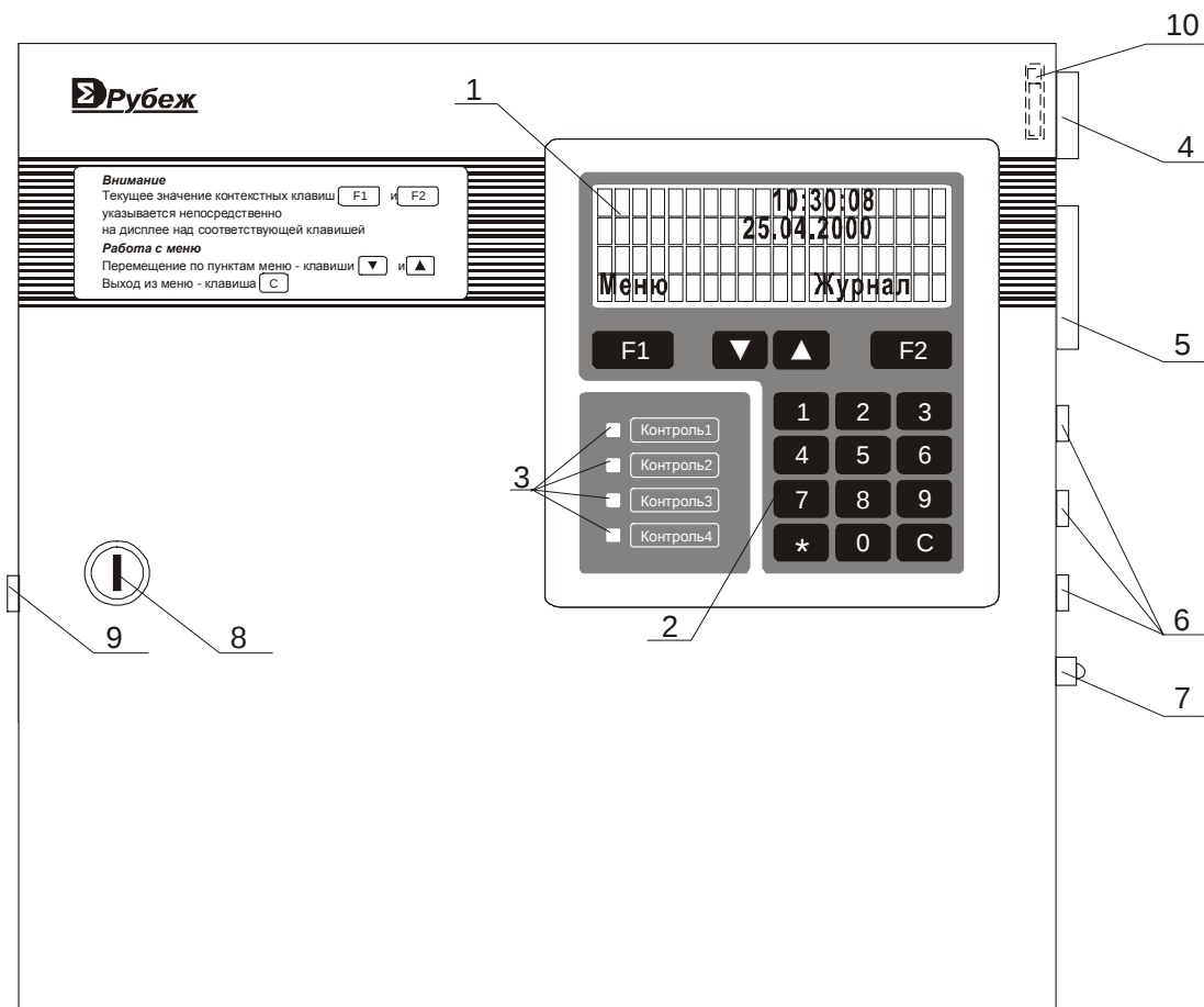
Рис. 8 Внешний вид БЦП исп.3
