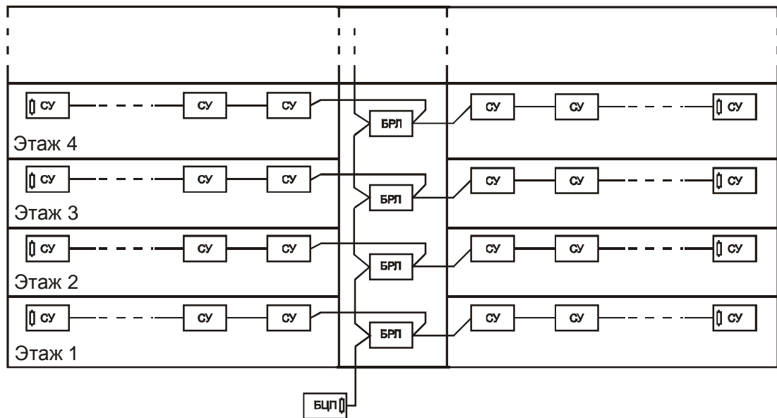
Рис. 16 Типовой вариант включения СУ
