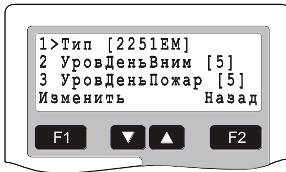
Рис. 23 Конфигурирование датчиков
