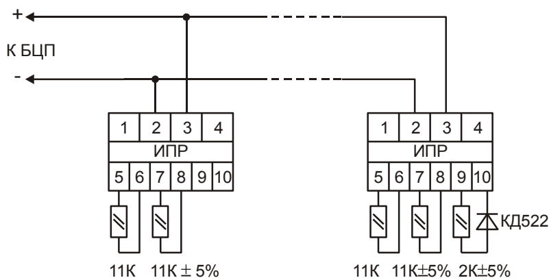
Рис. 17 Схема включения ручных ИП (ИПР и т. п.)
