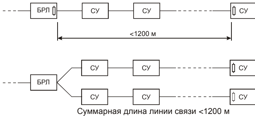
Рис. 5 Варианты включения СУ после БРЛ-03
