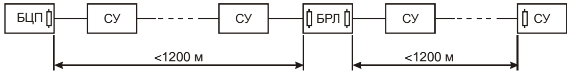
Рис. 3 Использование БРЛ-03 для удлинения линии связи
